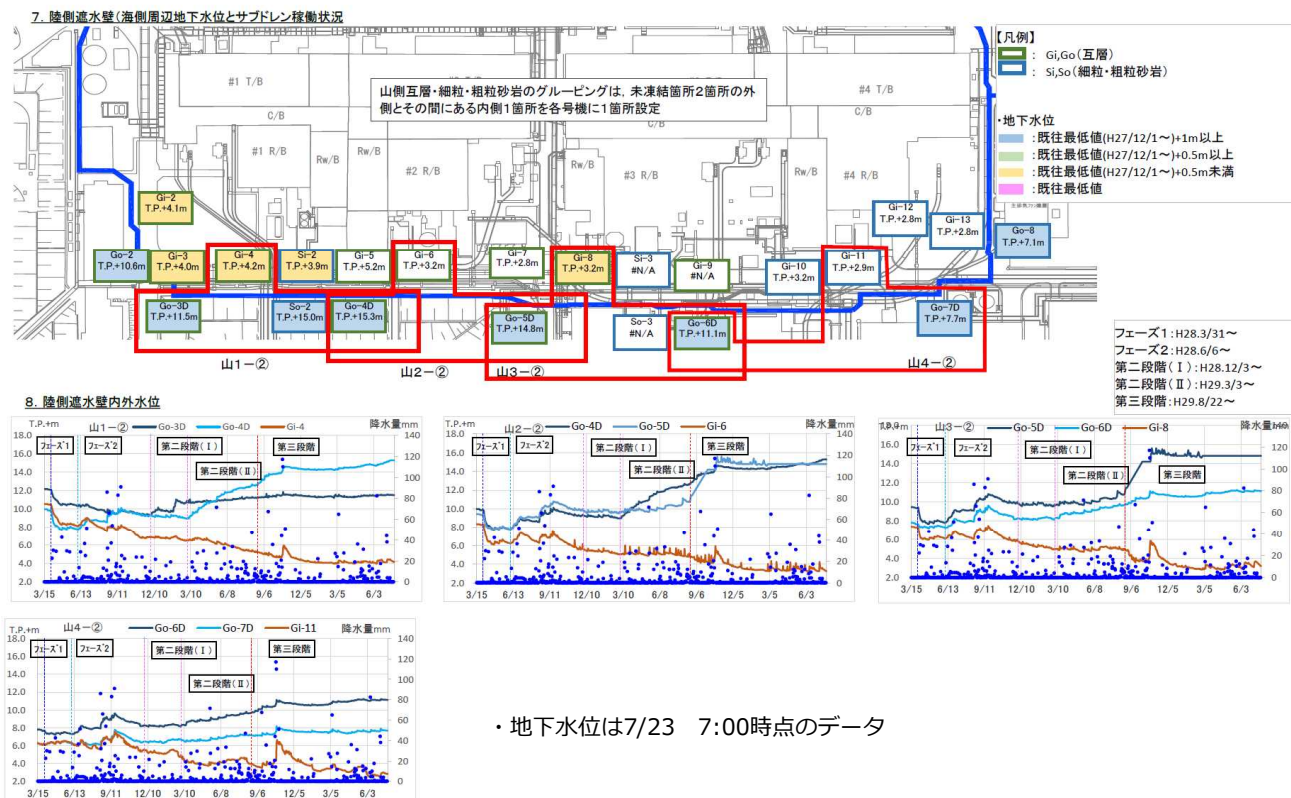
陸側遮水壁運用における監視項目（山側 互層・細粒・粗粒砂岩層水位）
