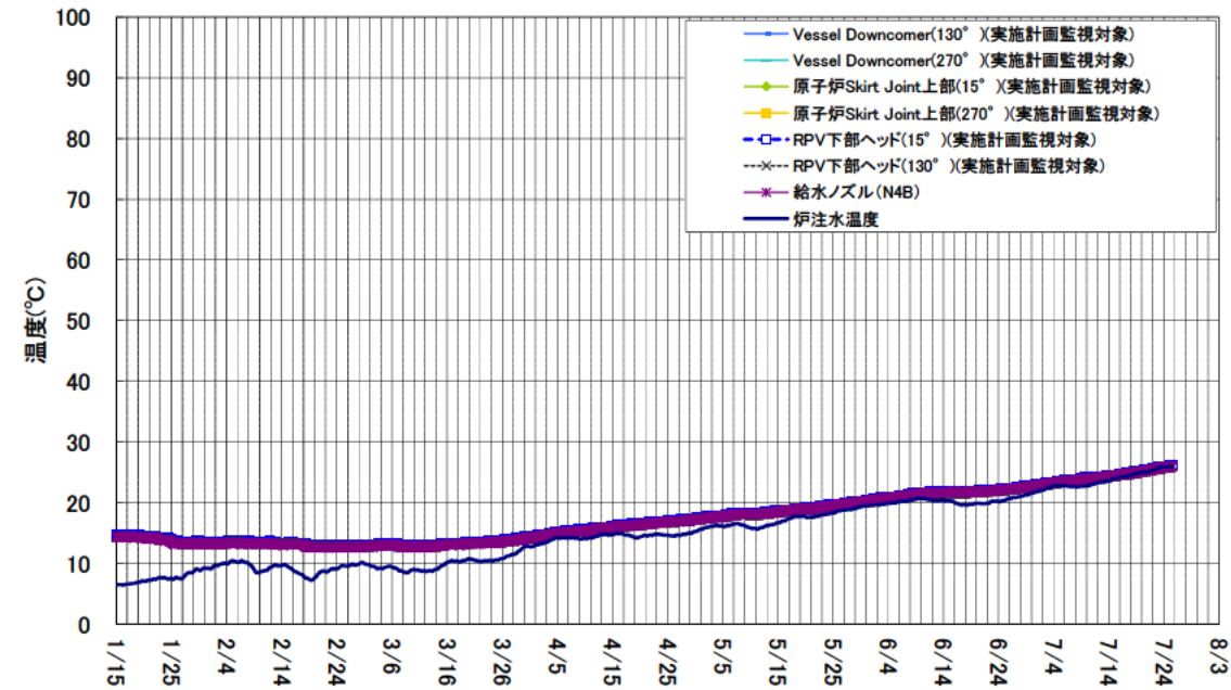
1号機 原子炉圧力容器まわり温度(1/15~7/25)
