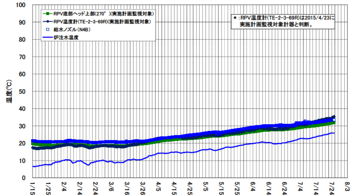
2号機 原子炉压力容器まわり温度(1/15~7/25)
