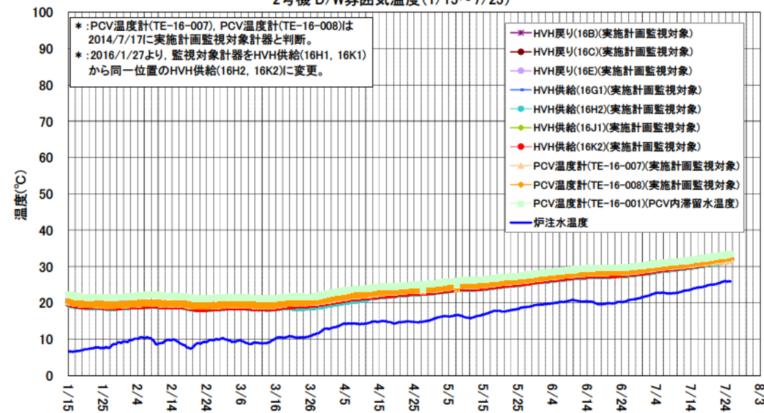
2号機 D/W雰囲気温度(1/15~7/25)
