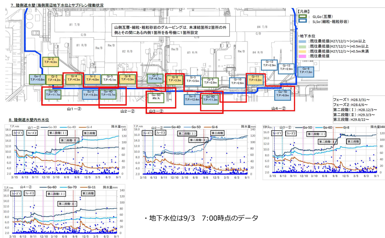
陸側遮水壁運用における監視項目（山側 互層・細粒・粗粒砂岩層水頭）
