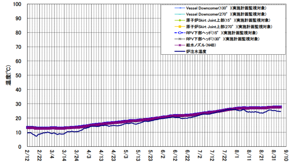
1号機 原子炉圧力容器まわり温度(2/12~9/5)
