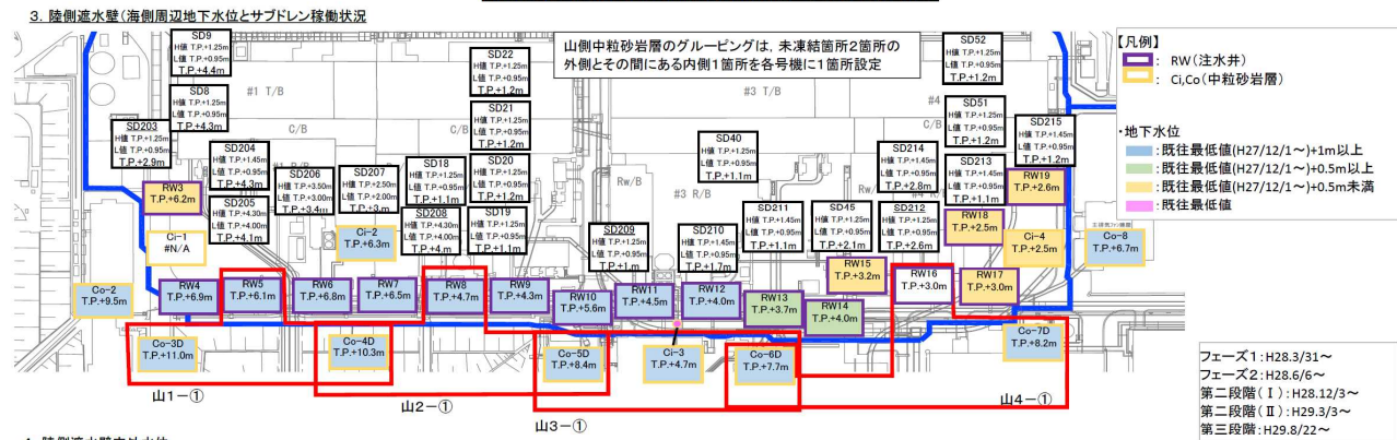
陸側遮水壁運用における監視項目(山側 中粒砂岩層水位)
