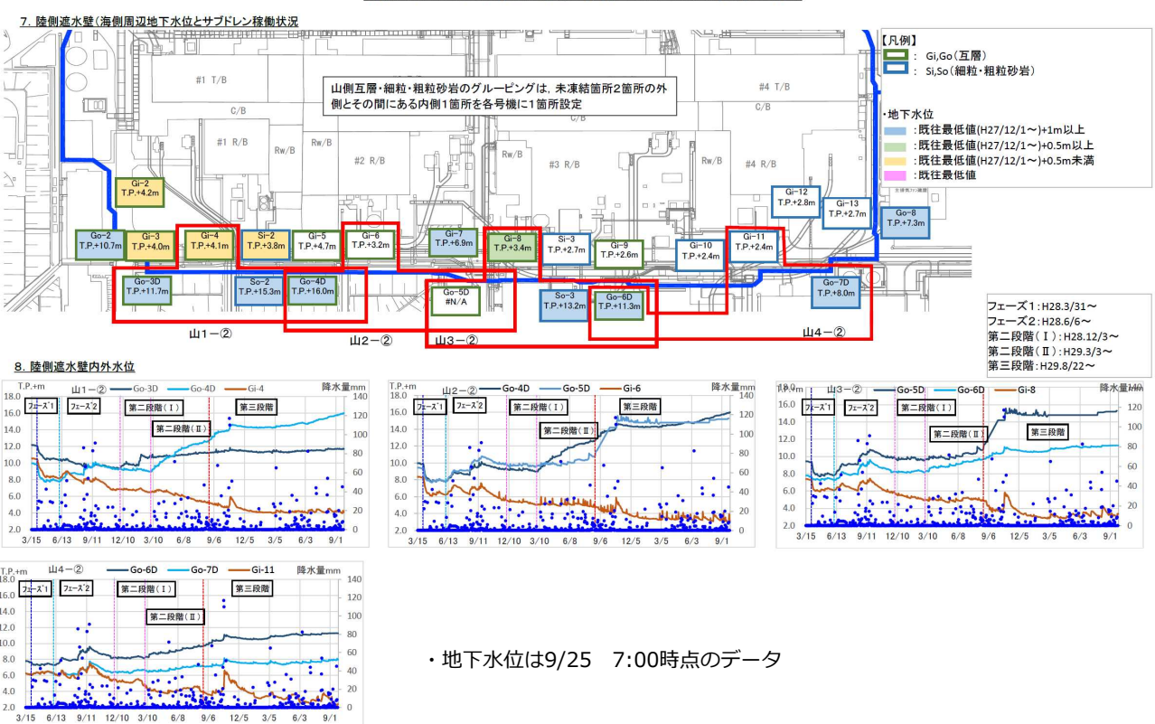
陸側遮水壁運用における監視項目(山側 互層・細粒・粗粒砂岩水位)
