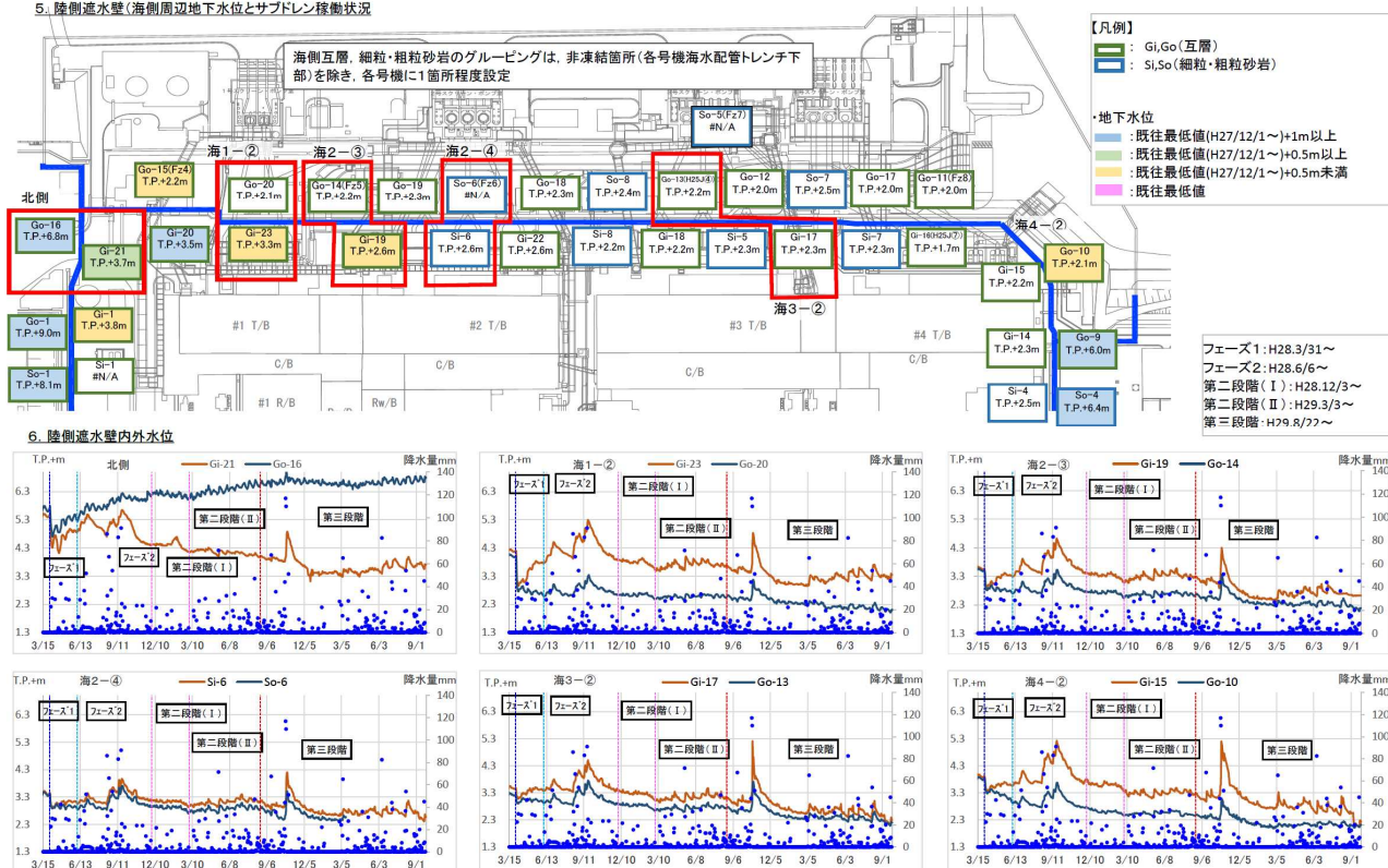
陸側遮水壁運用における監視項目(海側 互層・細粒・粗粒砂岩層水位)
