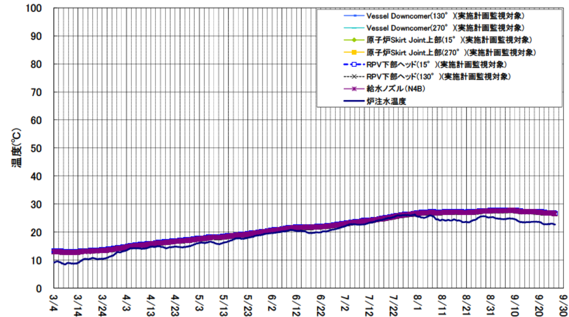
1号機 原子炉圧力容器まわり温度(3/4~9/26)
