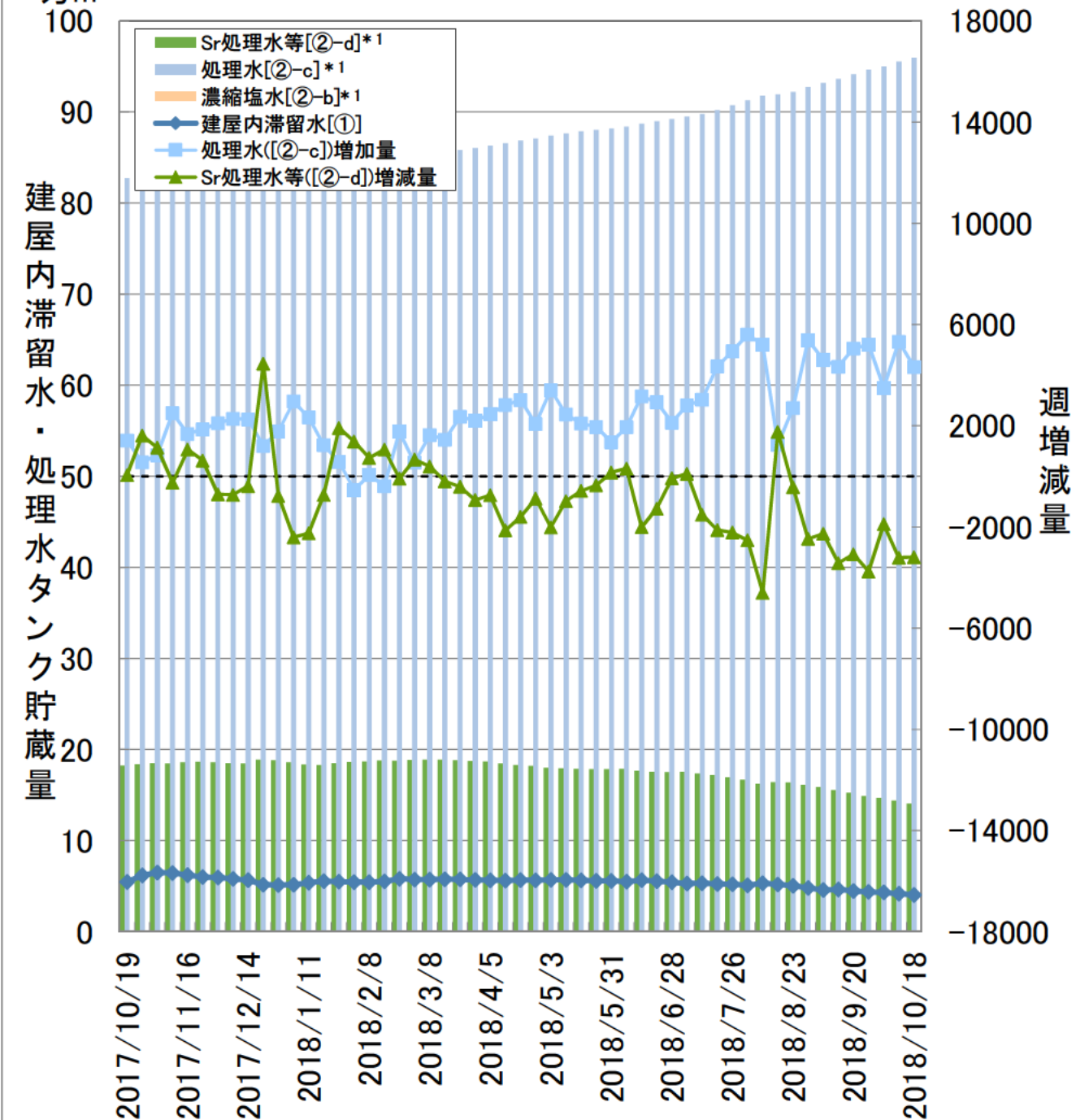
万m³ 建屋内滞留水、濃縮塩水及び処理水、Sr処理水等の推移m³/週
