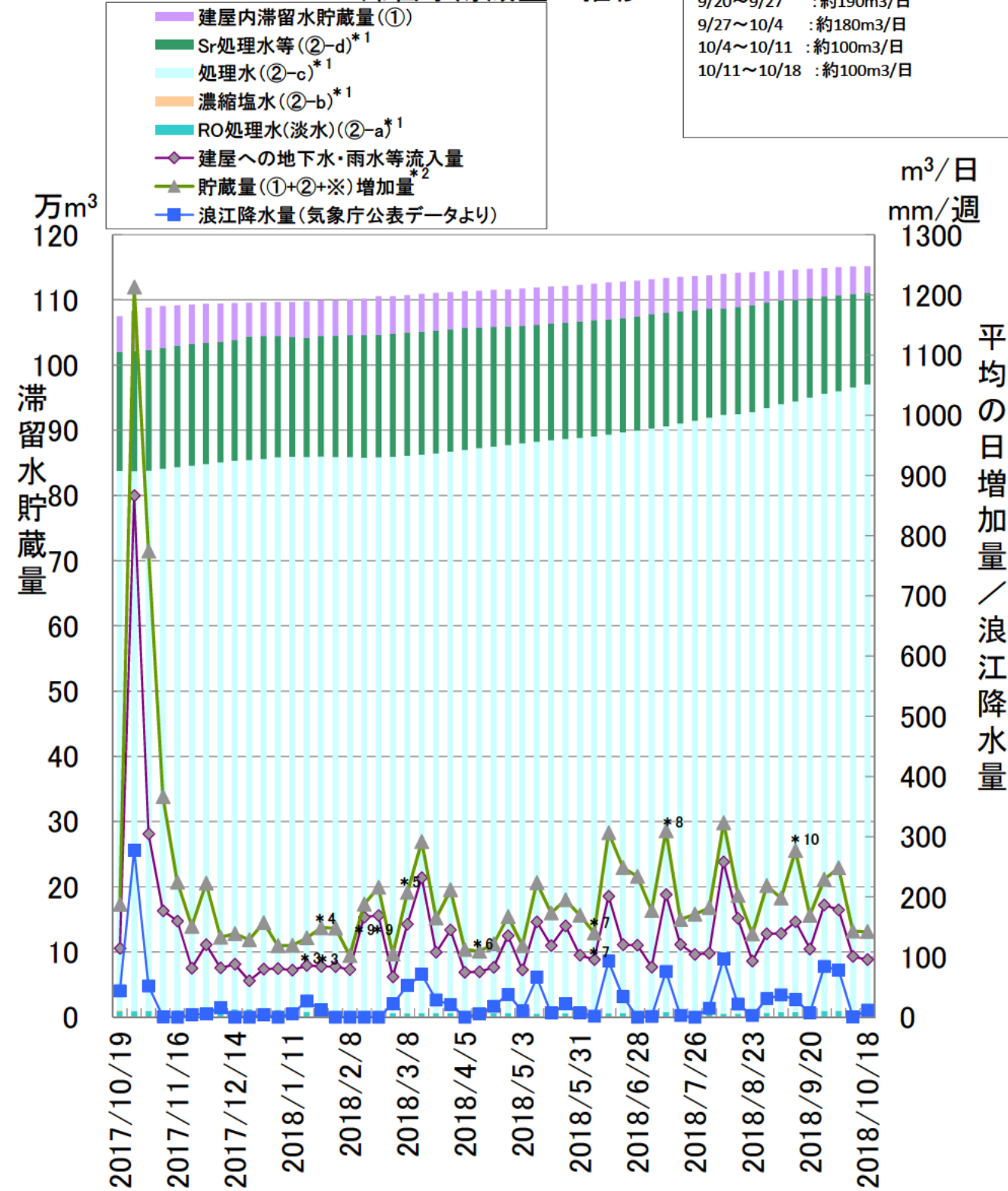
滞留水貯蔵量の推移
