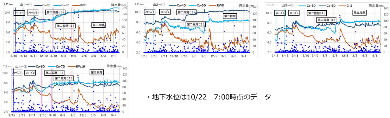
4. 陸側遮水壁内外水位
