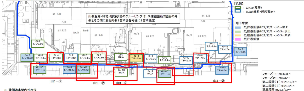
8. 陸側遮水壁内外水位
