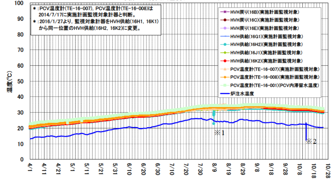
2号機 D/W雰囲気温度 (4/1~10/24)
