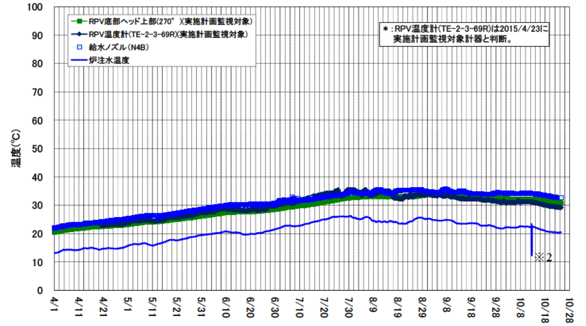
2号機 原子炉压力容器まわり温度 (4/1~10/24)
