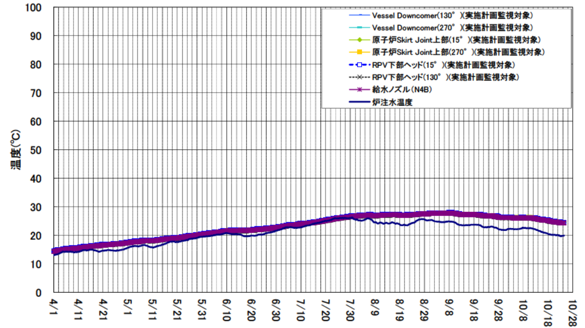
1号機 原子炉压力容器まわり温度 (4/1～10/24)
