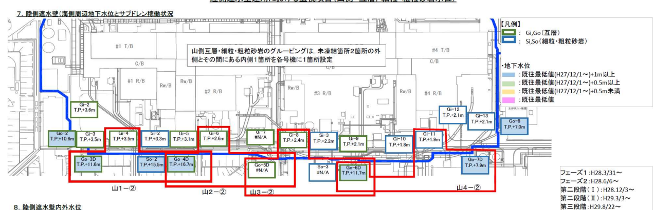
陸側遮水壁運用における監視項目（山側 互層、細粒・粗粒砂岩層水位）
