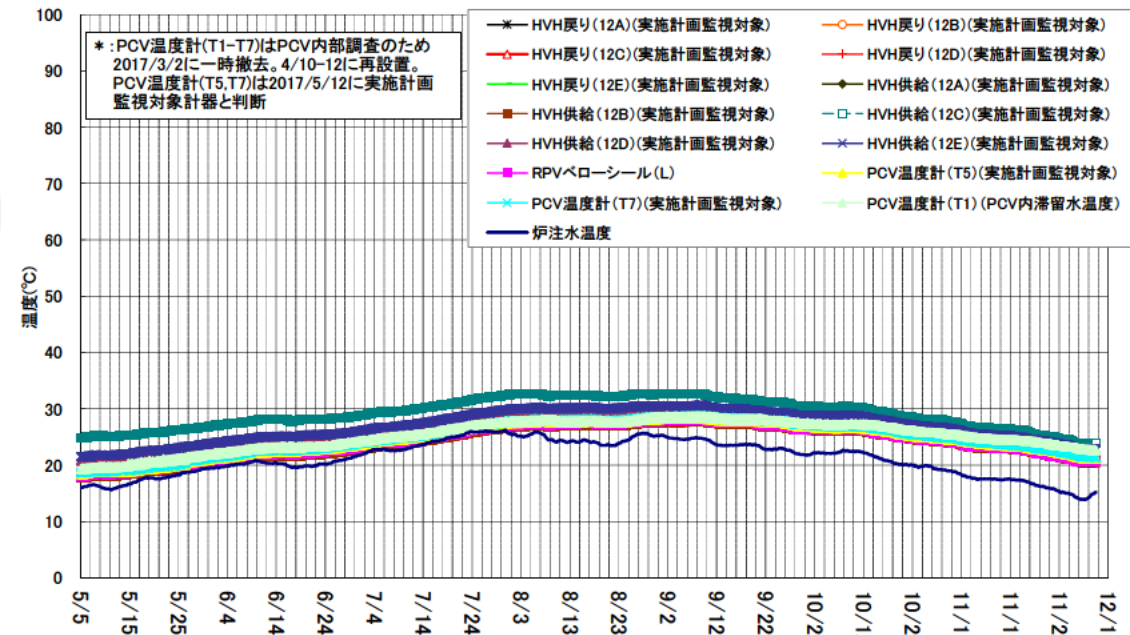
1号機 D/W雰囲気温度(5/5~11/28)
