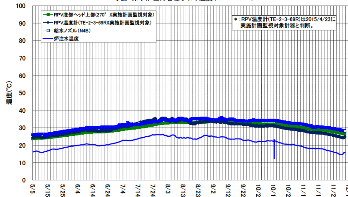
2号機 原子炉圧力容器まわり温度(5/5～11/28)
