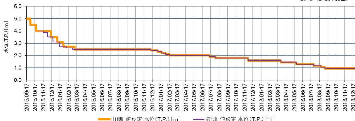
山側・海側サブドレン（L値設定）
