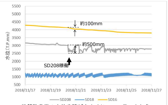
【地盤改良後】No.208水位低下量の20%
