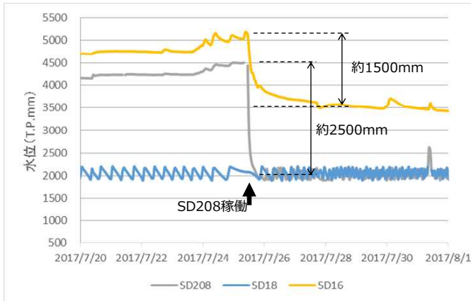
【地盤改良前】No.208水位低下量の60%
