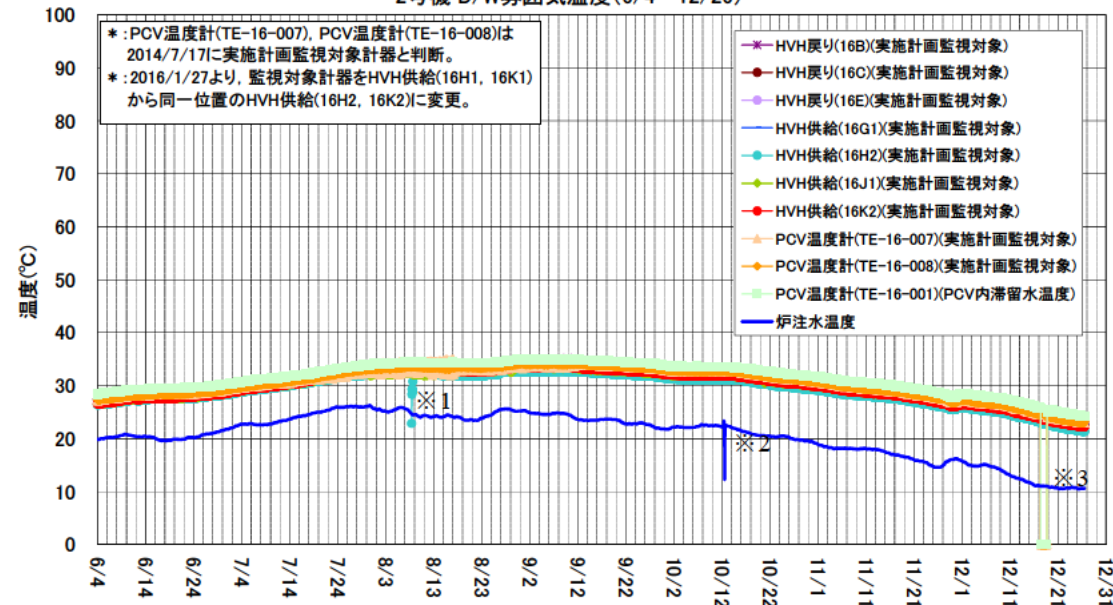
2号機 D/W雰囲気温度(6/4~12/26)
