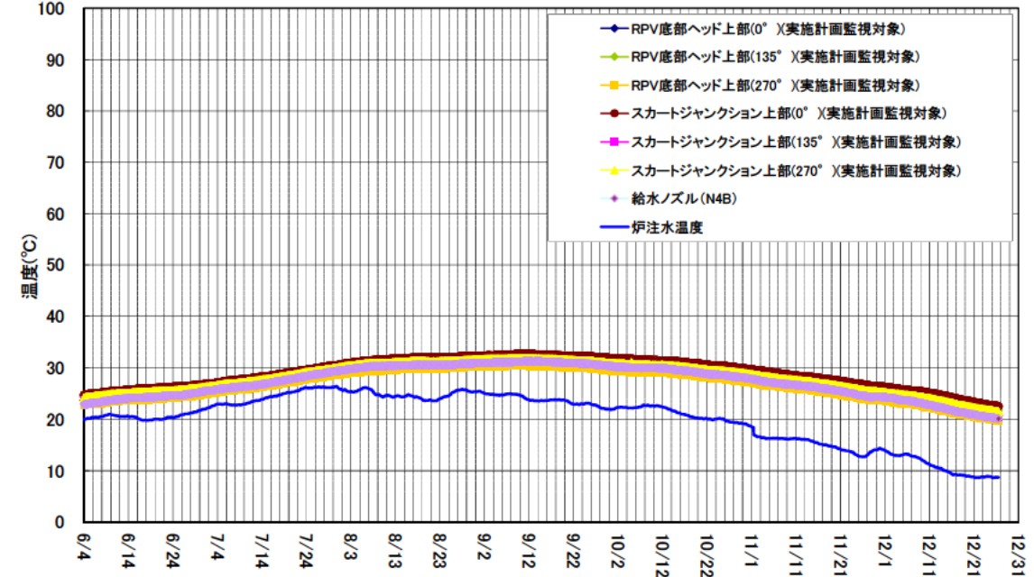
3号機 原子炉圧力容器まわり温度 (6/4~12/26)
