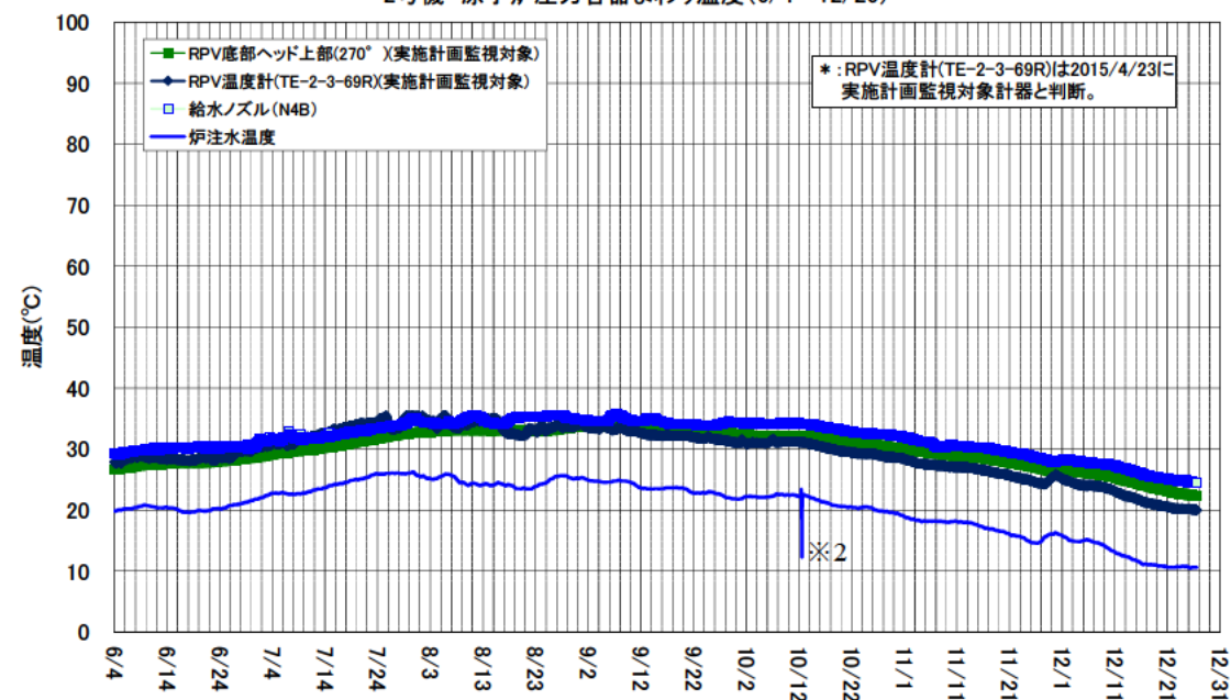
2号機 原子炉圧力容器まわり温度(6/4~12/26)
