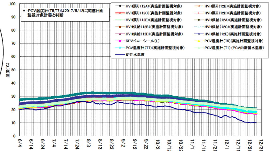
1号機 D/W雰囲気温度(6/4~12/26)
