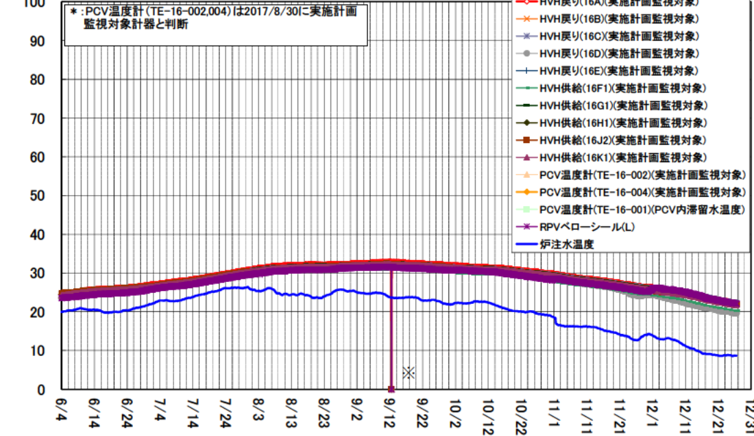
3号機 D/W雰囲気温度 (6/4~12/26)
