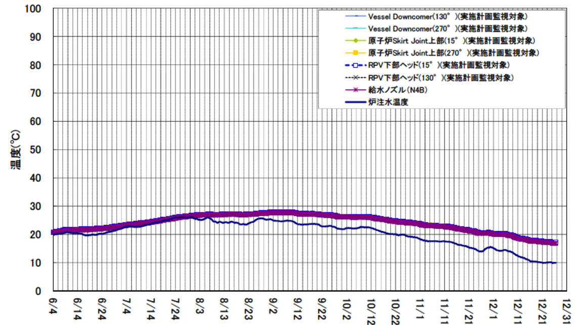
1号機 原子炉圧力容器まわり温度(6/4~12/26)
