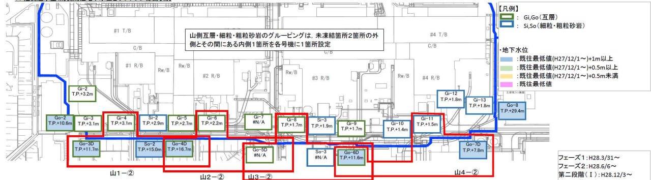
陸側遮水壁運用における監視項目(山側 互層、細粒・粗粒砂岩層水位)
