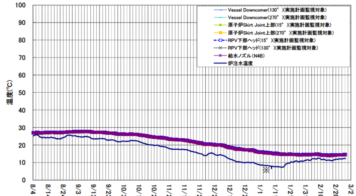
1号機 原子炉圧力容器まわり温度(8/4~2/26)
