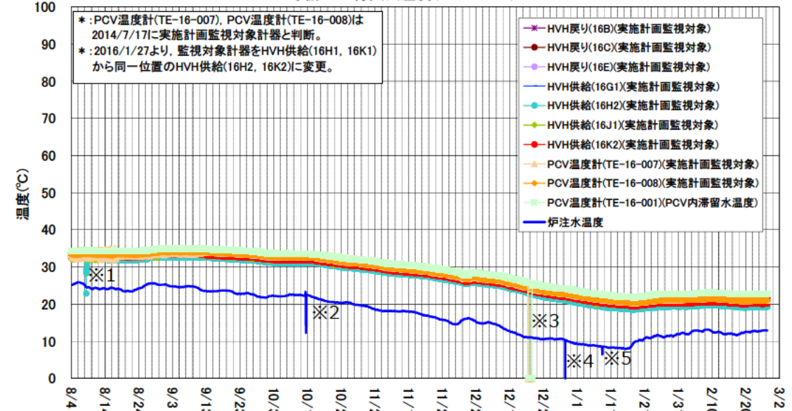
2号機 D/W雰囲気温度(8/4~2/26)
