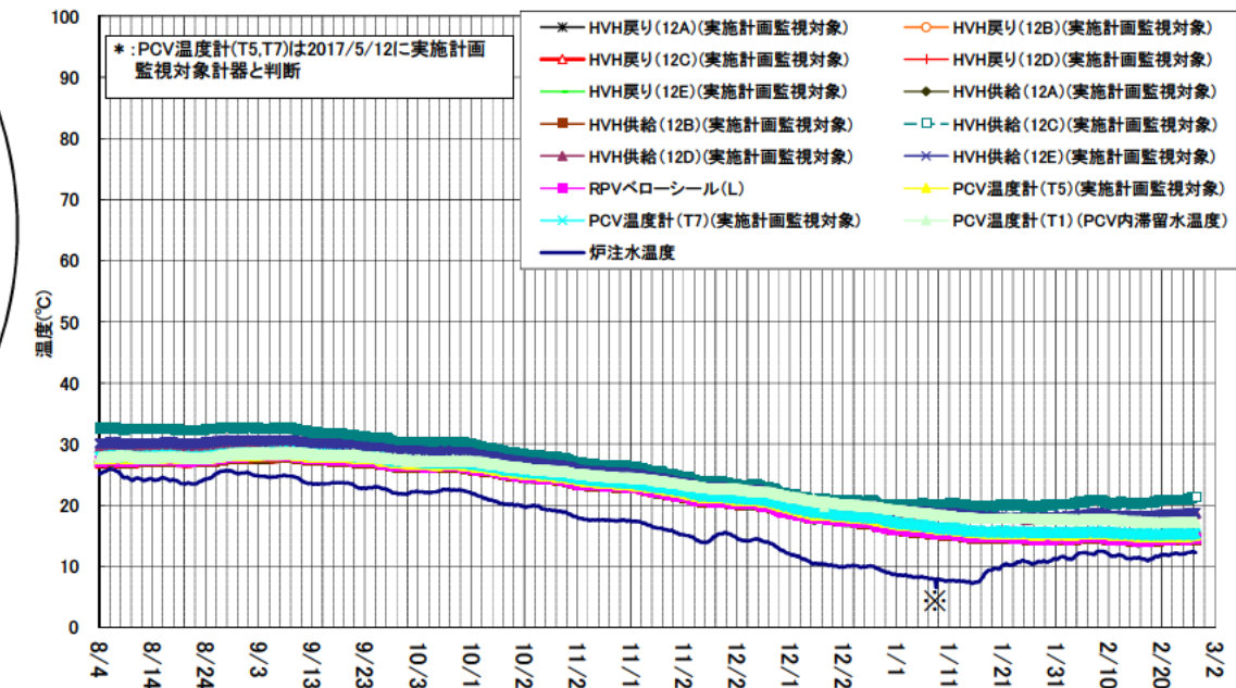
1号機 D/W雰囲気温度(8/4~2/26)
