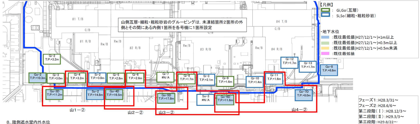
陸側遮水壁運用における監視項目（山側 互層、細粒・粗粒砂岩層水位）
