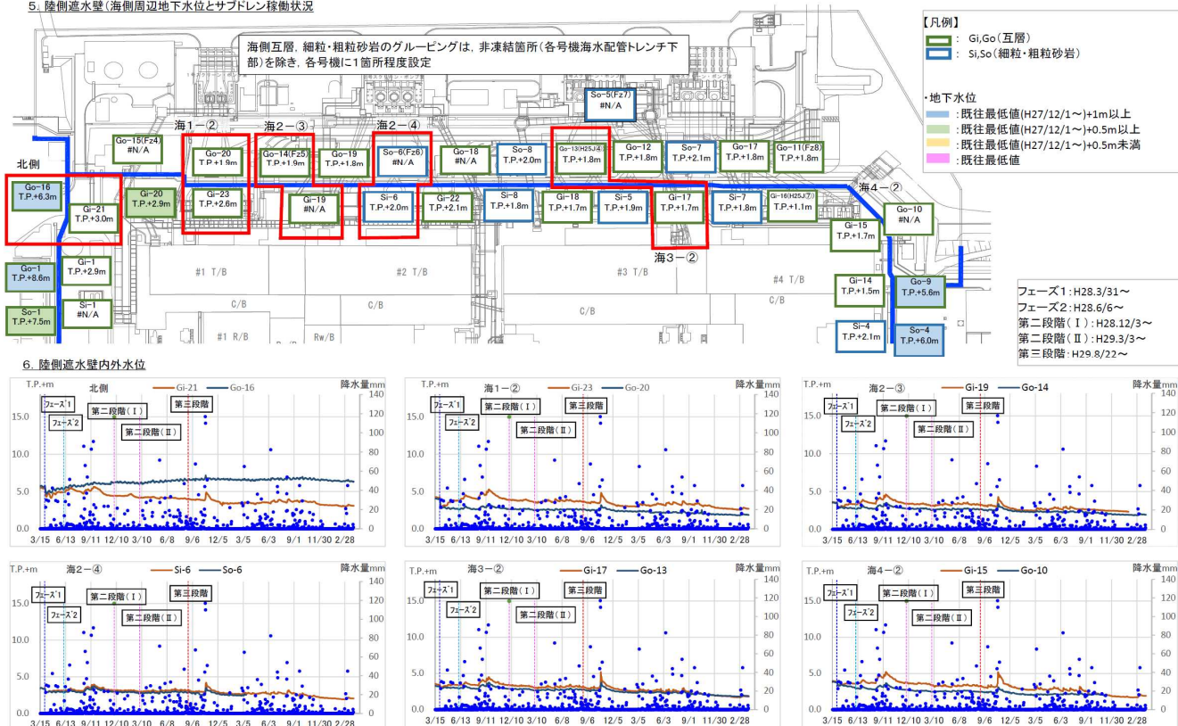
陸側遮水壁運用における監視項目（海側 互層、細粒・粗粒砂岩水位）
