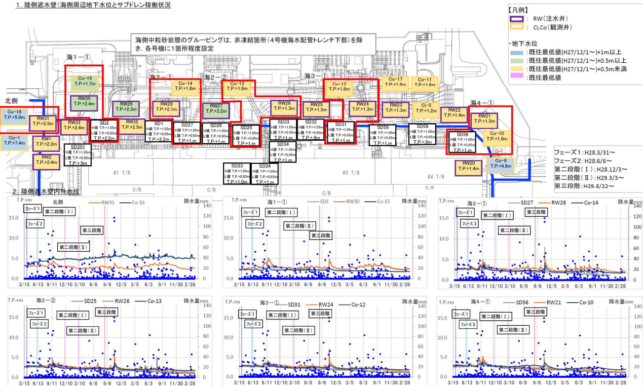
1. 陸側遮水壁（海側周辺地下水位とサブドレン稼働状況）
