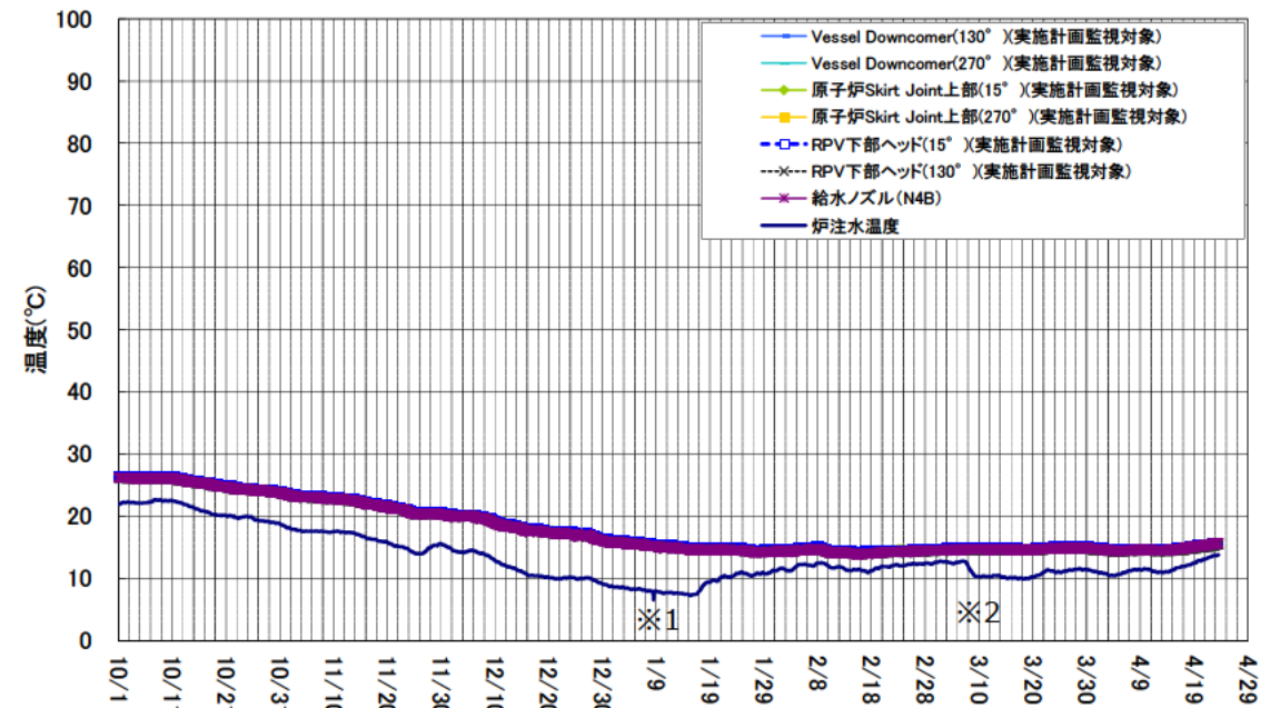
1号機 原子炉圧力容器まわり温度(10/1~4/23)
