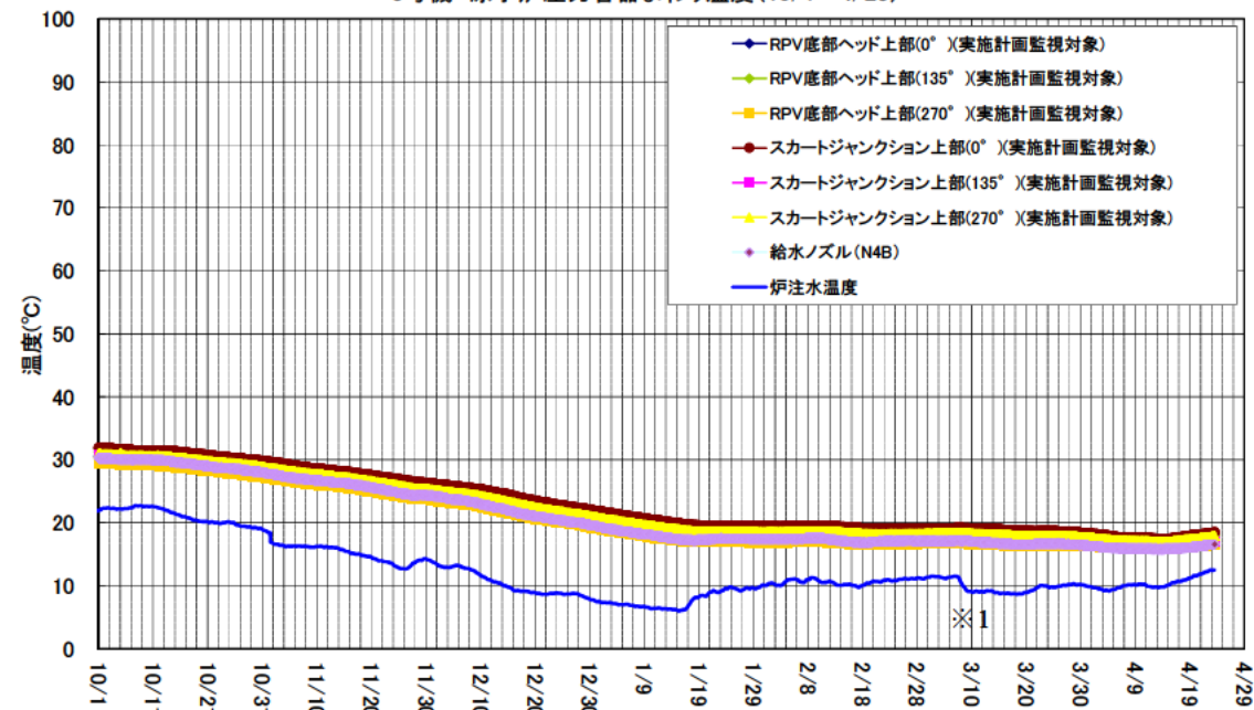
3号機 原子炉圧力容器まわり温度(10/1~4/23)
