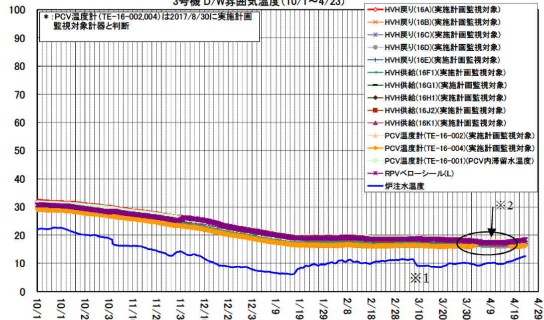
3号機 D/W雰囲気温度(10/1~4/23)
