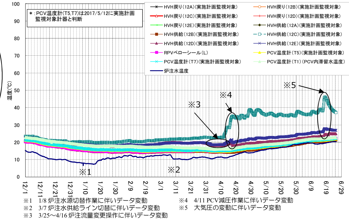
1号機 D/W雰囲気温度(12/1~6/25)
