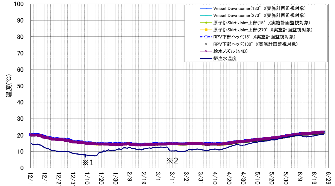
1号機 原子炉压力容器まわり温度(12/1~6/25)
