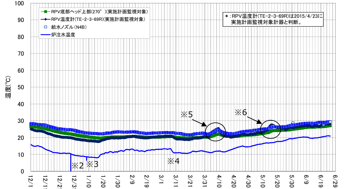
2号機 原子炉压力容器まわり温度 (12/1~6/25)
