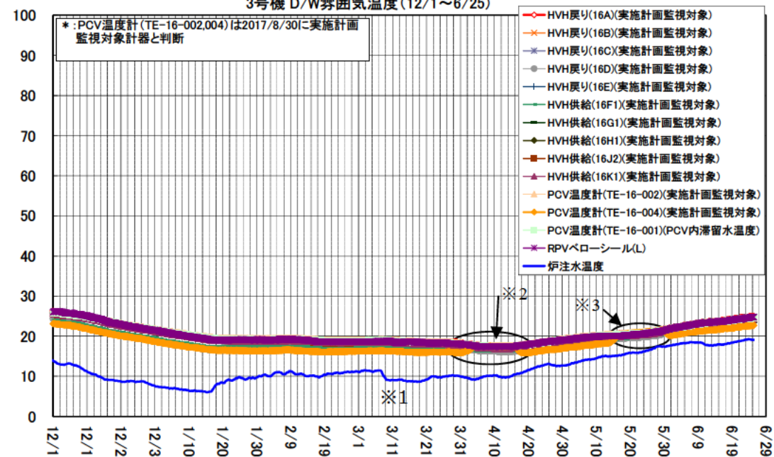
3号機 D/W雰囲気温度(12/1～6/25)
