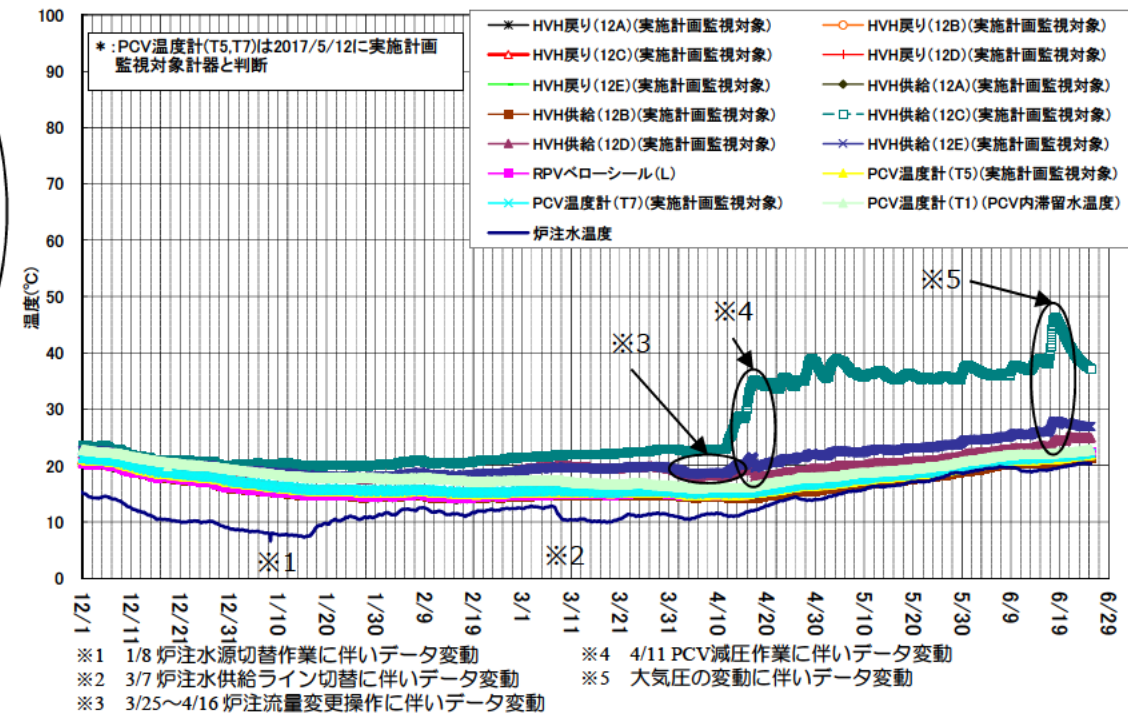
1号機 D/W雰囲気温度(12/1~6/25)
