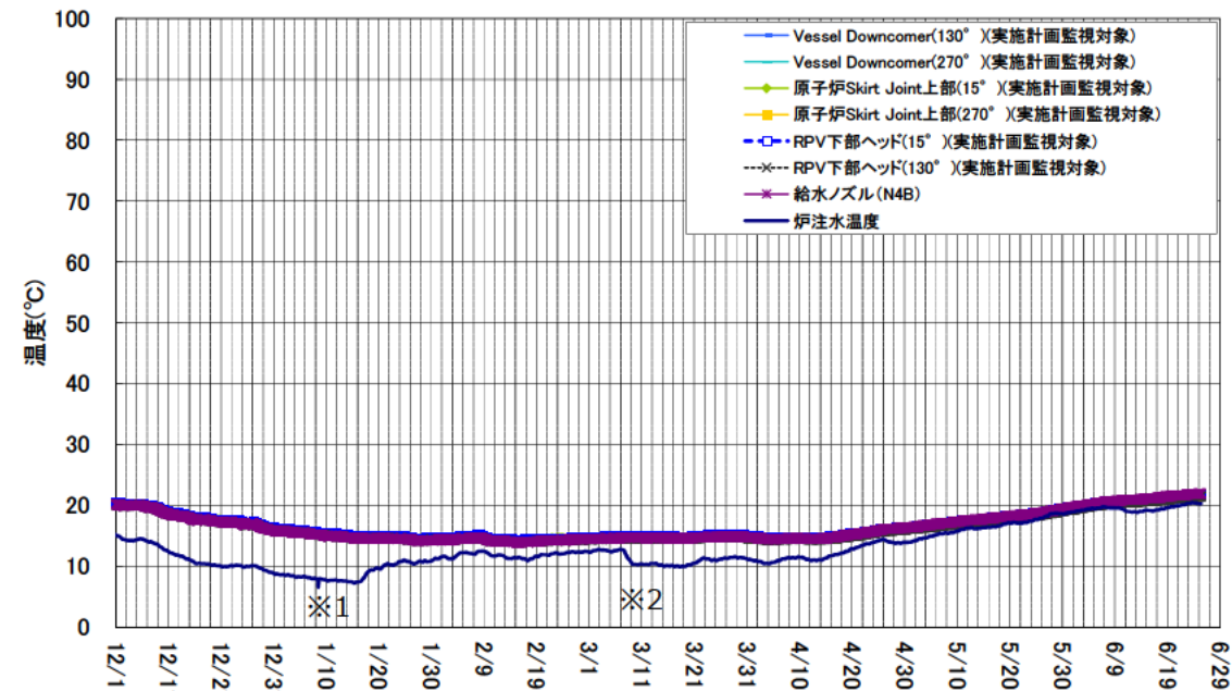
1号機 原子炉圧力容器まわり温度(12/1~6/25)
