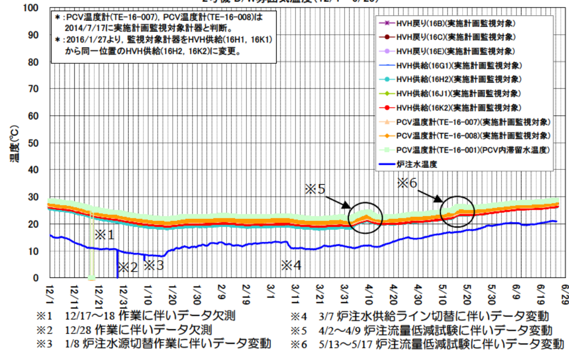
2号機 D/W雰囲気温度(12/1~6/25)
