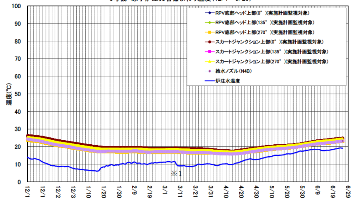
3号機 原子炉圧力容器まわり温度(12/1～6/25)
