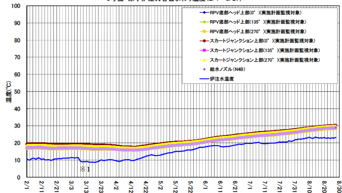
3号機 原子炉圧力容器まわり温度(2/1~8/27)
