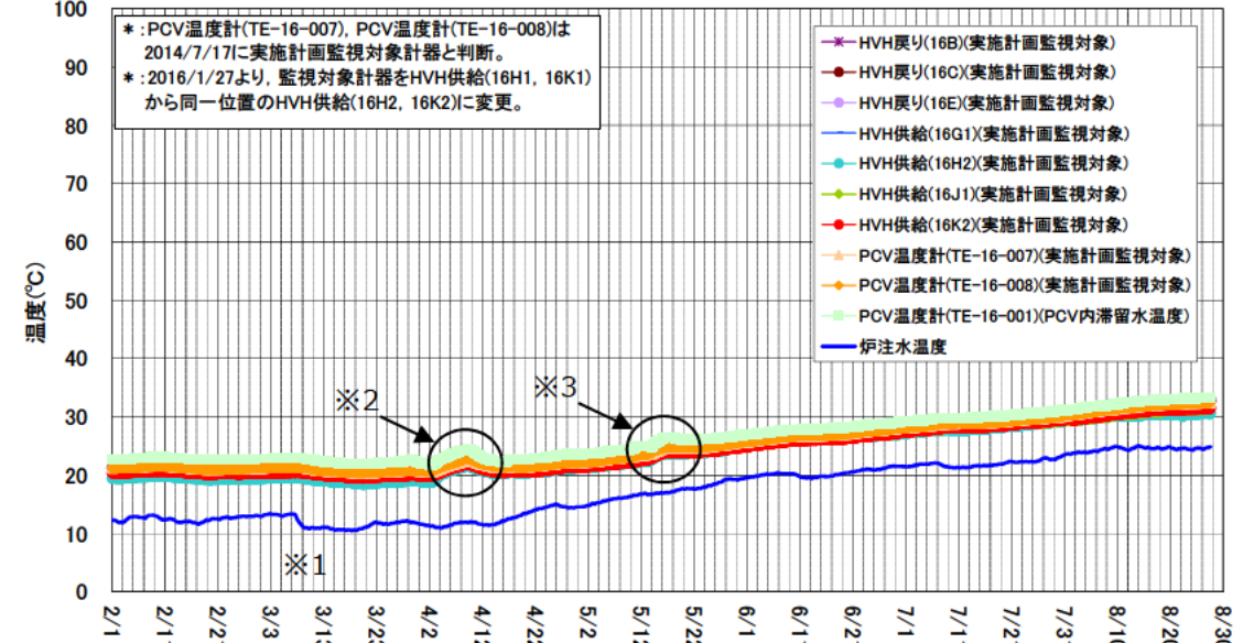
2号機 D/W雰囲気温度(2/1～8/27)
