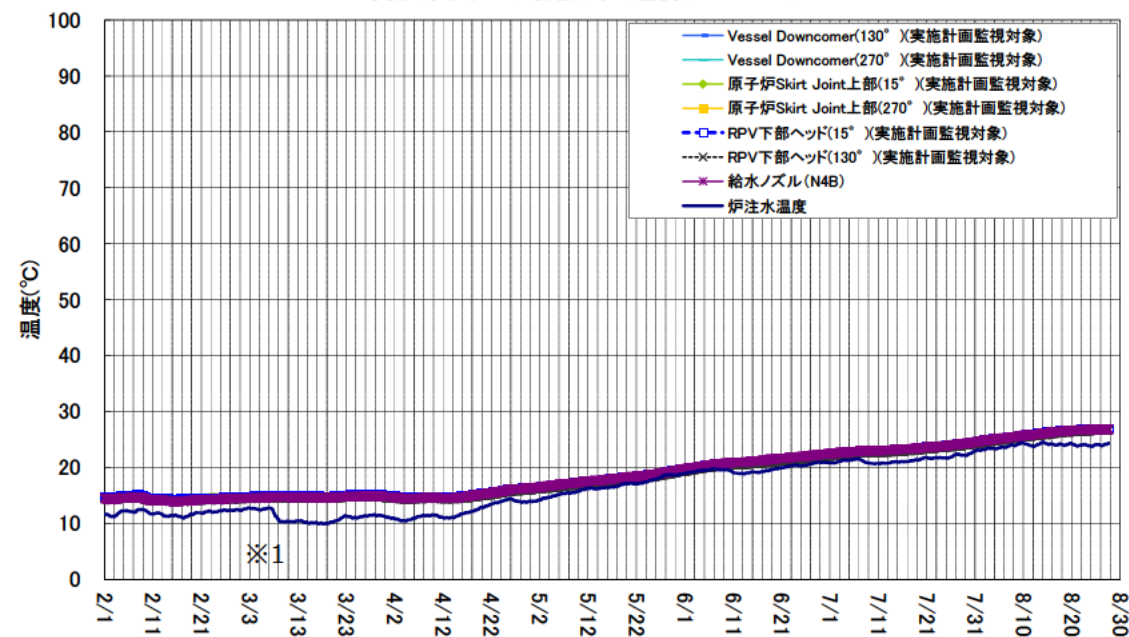
1号機 原子炉圧力容器まわり温度(2/1~8/27)
