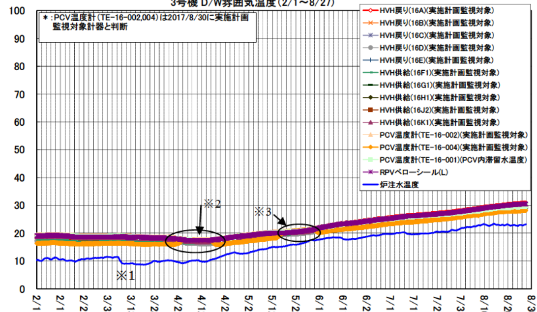
3号機 D/W雰囲気温度(2/1~8/27)
