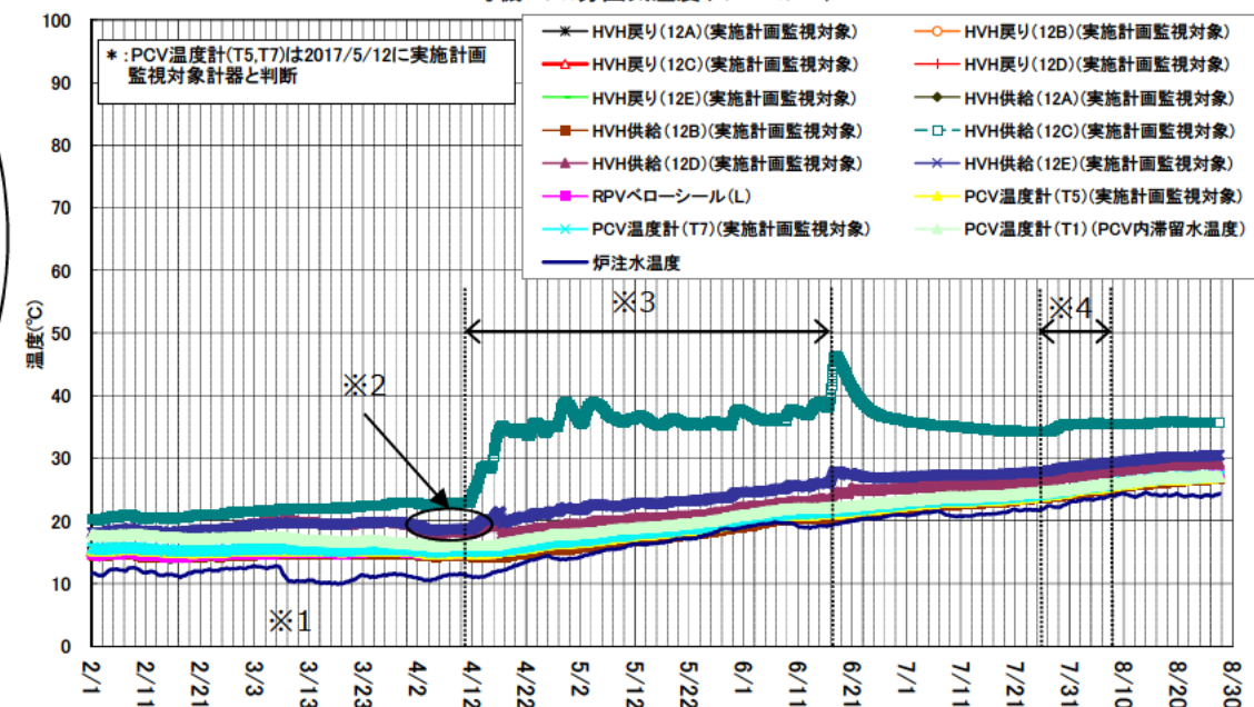
1号機 D/W雰囲気温度(2/1~8/27)
