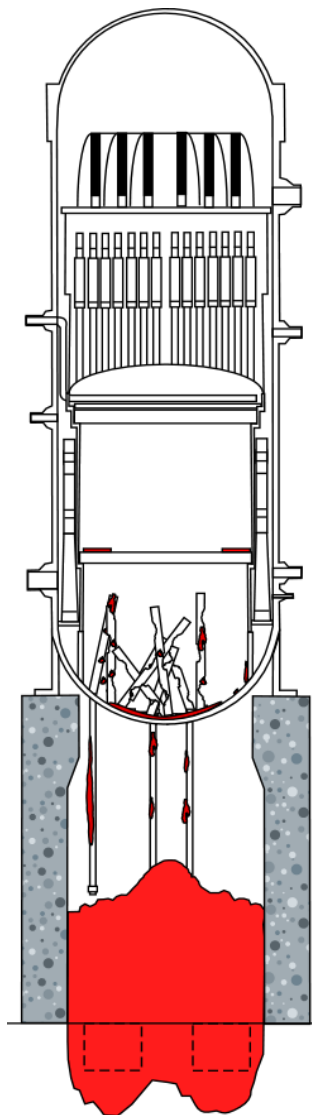
図 A8-2 1 号機の燃料デブリにおいて分析により確認する事項
