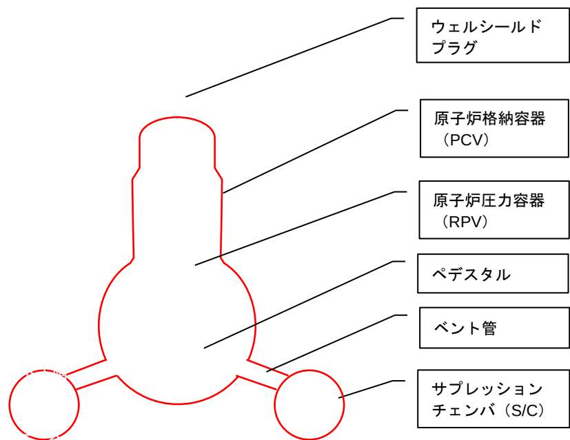
図 29 原子炉建屋内構造図
