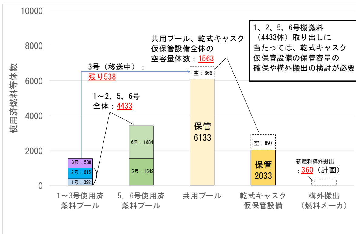
図18 使用済燃料等の保管状況（2019年8月29日現在）
