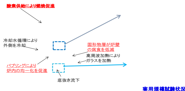
図7 コールドクルーシブル誘導加熱炉(CCIM)概要
