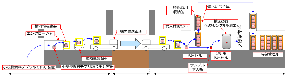
図7 燃料デブリの取り出し、収納・移送・保管のイメージ
