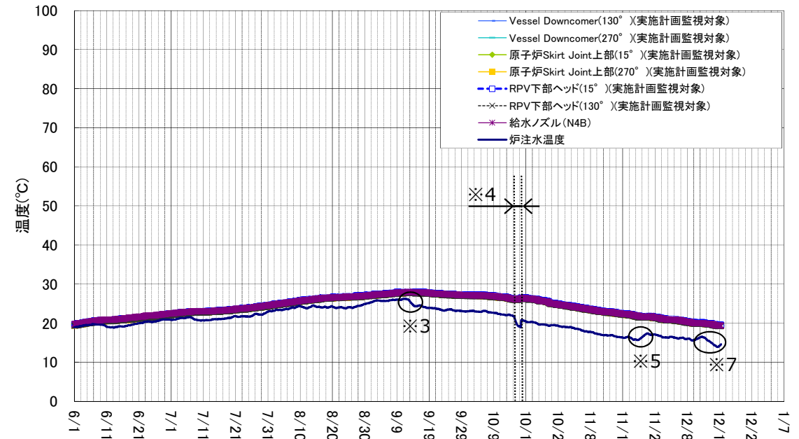
1号機 原子炉圧力容器まわり温度(6/1~12/18)
