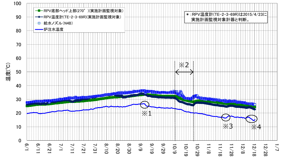
2号機 原子炉压力容器まわり温度 (6/1～12/18)
