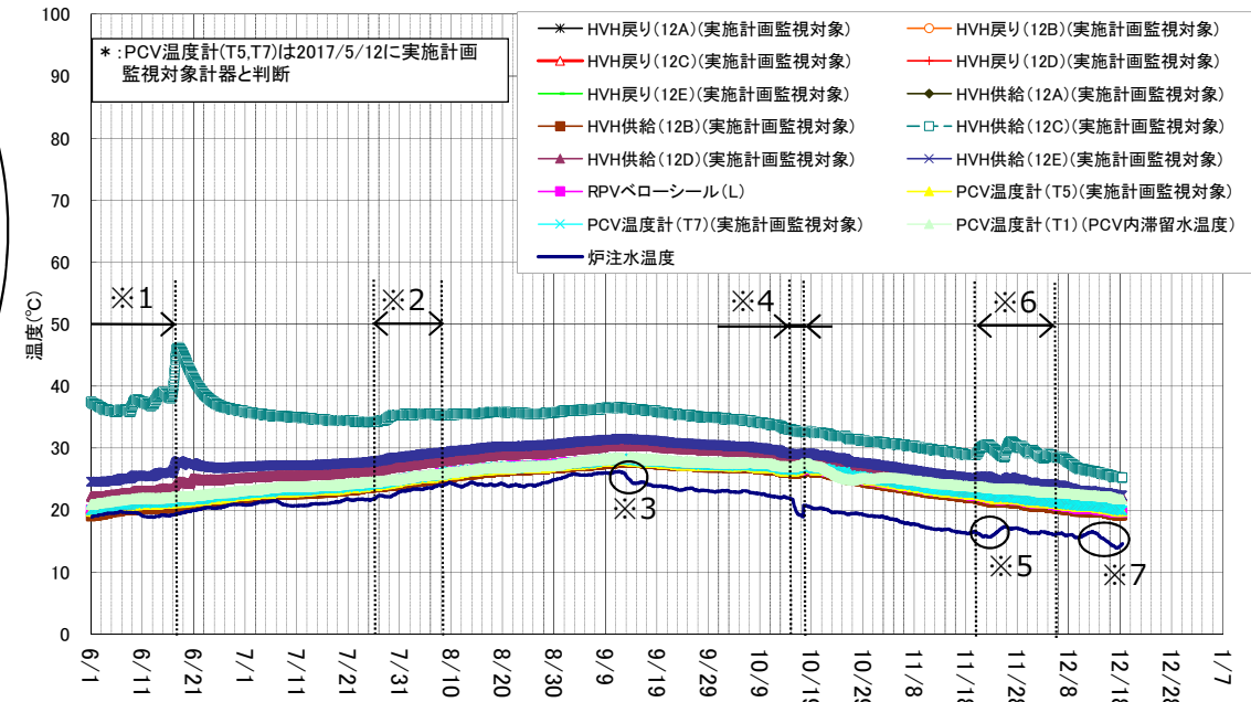
1号機 D/W雰囲気温度(6/1~12/18)
