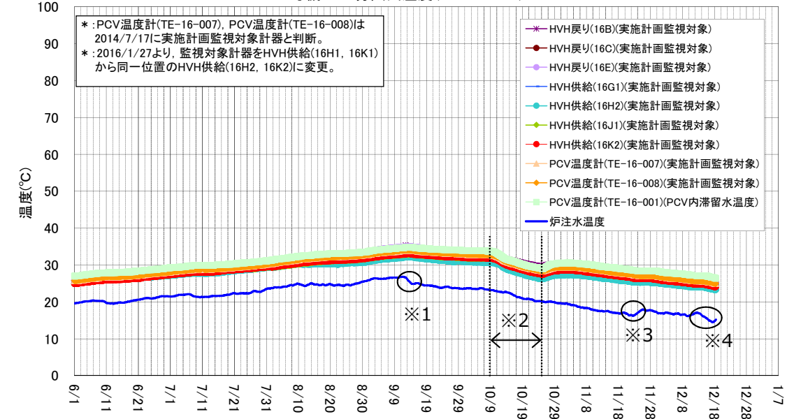
2号機 D/W雰囲気温度 (6/1～12/18)
