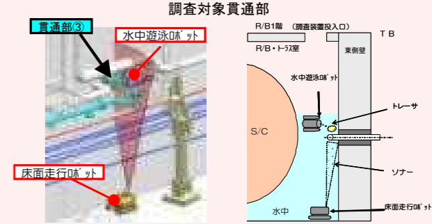
トラス室東側断面調査イメージ
