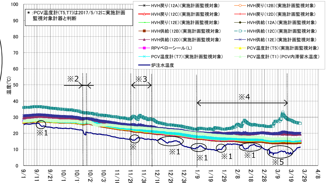
1号機 D/W雰囲気温度(9/1~3/25)
