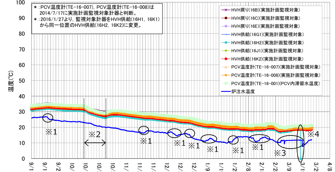
2号機 D/W雰囲気温度(9/1～3/25)
