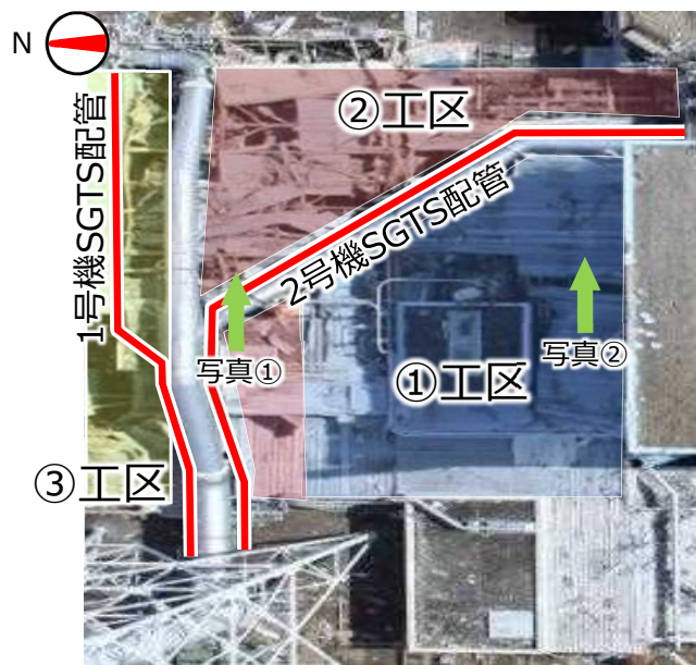
【図3】作業工区割図
