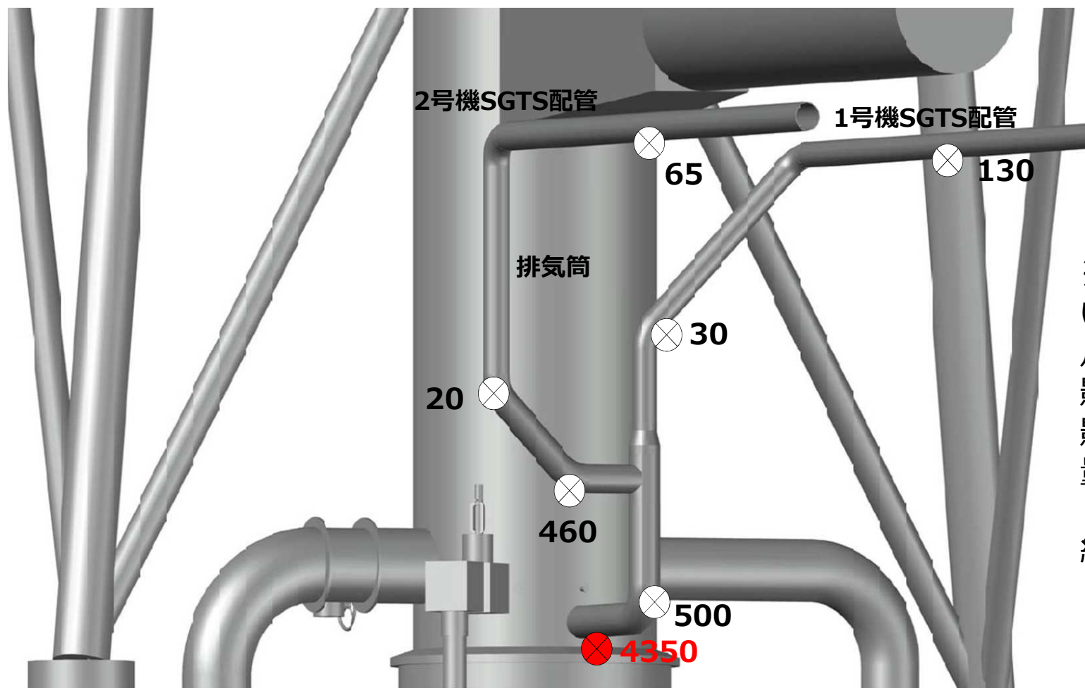
測定箇所図
