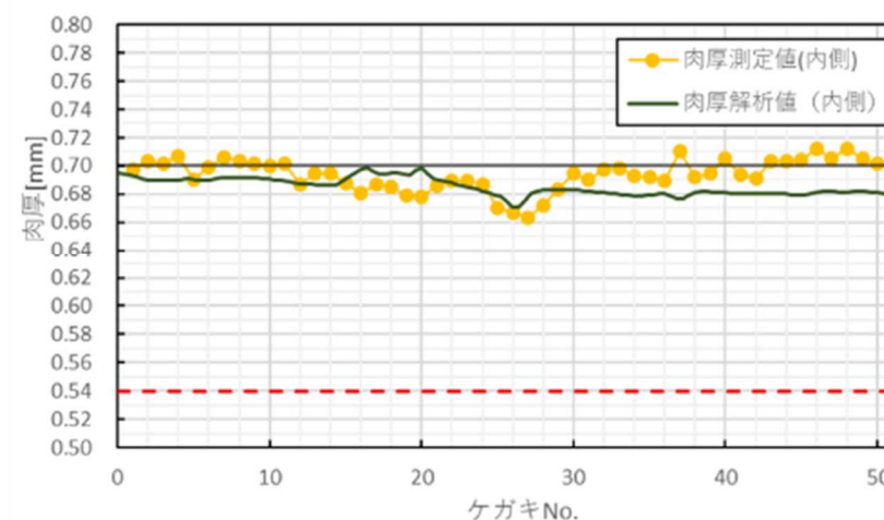
模擬棒（曲率内側）曲げ戻し後の被覆管肉厚
