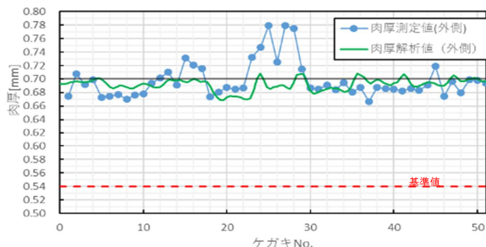
模擬棒（曲率外側）曲げ戻し後の被覆管肉厚
