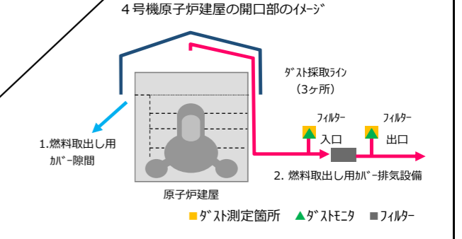
4号機原子炉建屋の開口部のイメージ ダスト採取ライン(3ヶ所) 月間平均値が一番高い箇所の ダストモニタの値を②に採用
