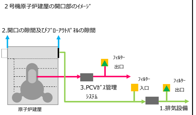
2号機原子炉建屋の開口部のイメージ 2.開口の隙間及び燃料取出し用カバーの隙間 月間平均値が一番高い箇所の ダストモニタの値を②に採用
