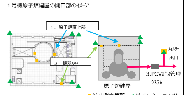
1号機原子炉建屋の開口部のイメージ 月間平均値が一番高い箇所の ダストモニタの値を②に採用
