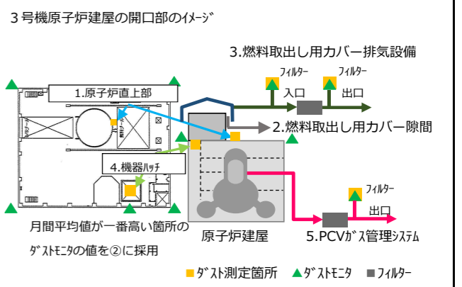
3号機原子炉建屋の開口部のイメージ 月間平均値が一番高い箇所の ダストモニタの値を②に採用
