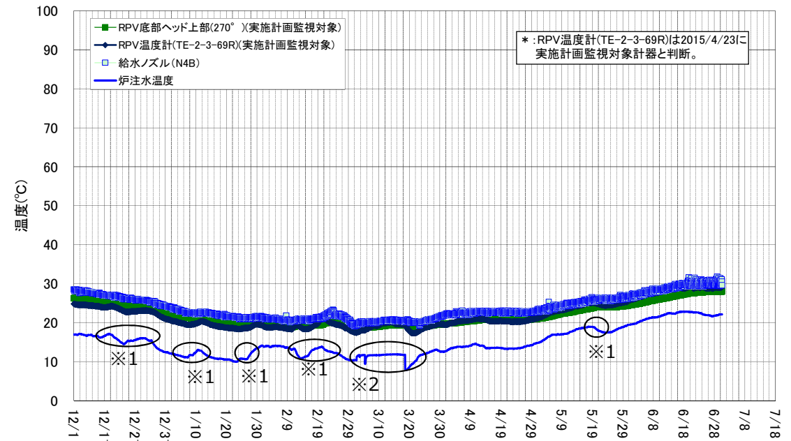
2号機 原子炉压力容器まわり温度(12/1～6/30)
