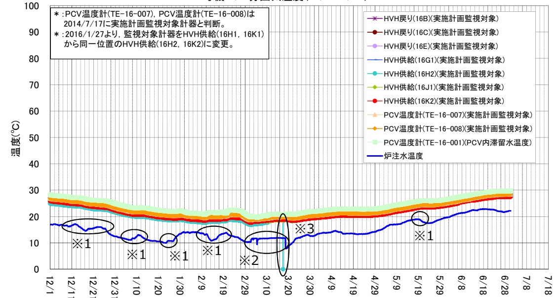
2号機 D/W雰囲気温度(12/1～6/30)
