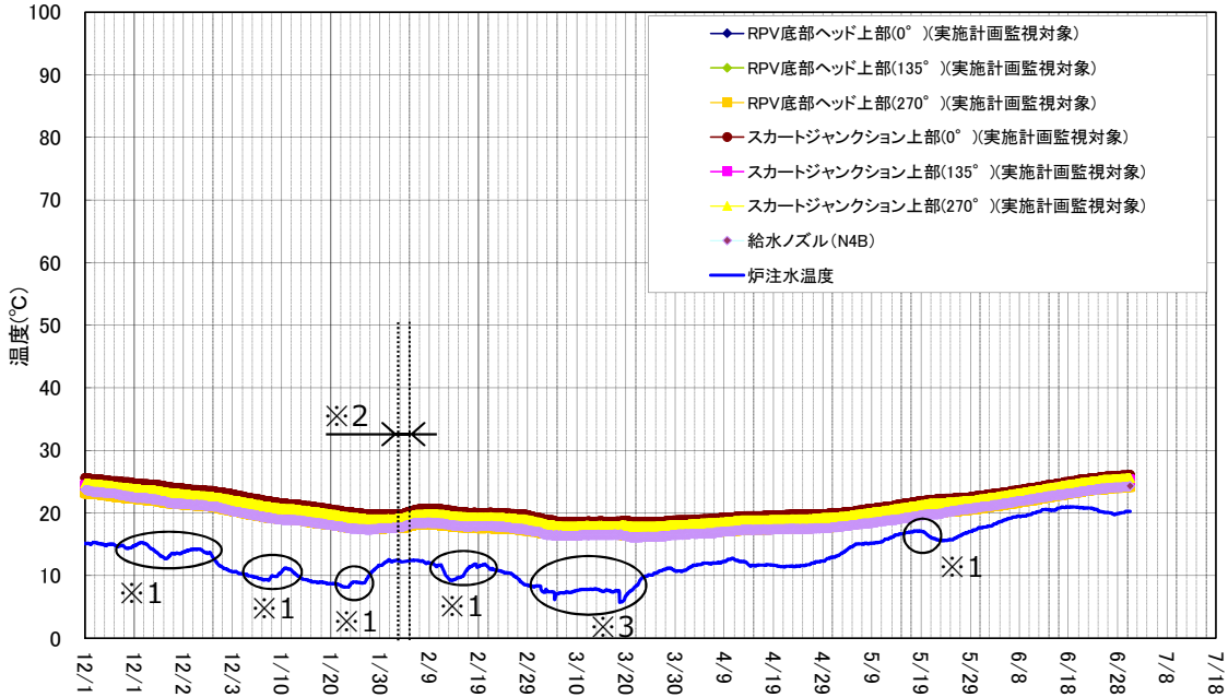
3号機 原子炉压力容器まわり温度(12/1～6/30)
