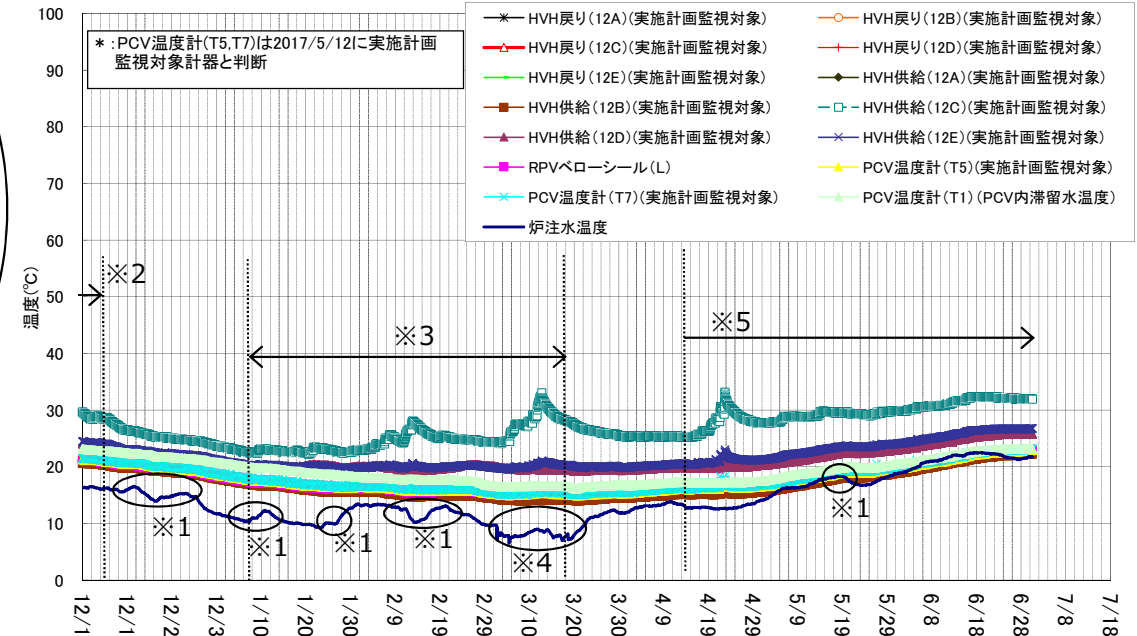
1号機 D/W雰囲気温度(12/1～6/30)
