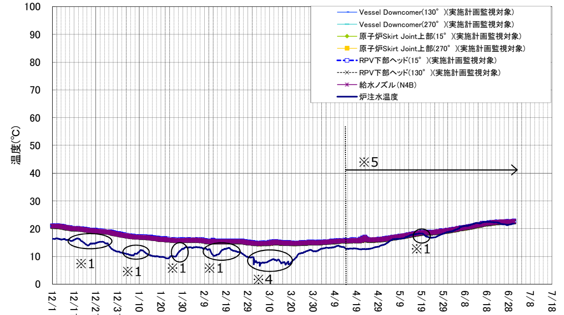
1号機 原子炉圧力容器まわり温度(12/1～6/30)
