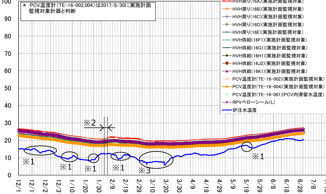
3号機 D/W雰囲気温度(12/1～6/30)
