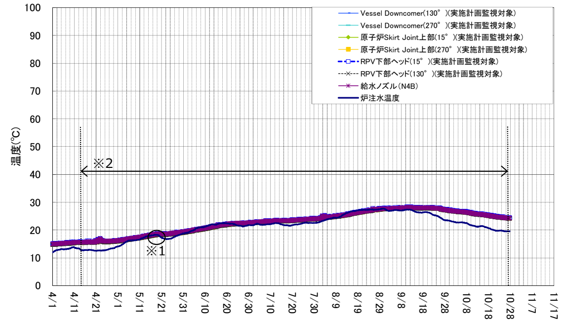
1号機 原子炉圧力容器まわり温度(4/1~10/27)
