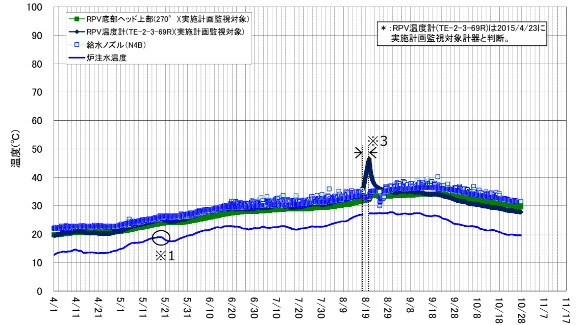
2号機 原子炉压力容器まわり温度(4/1～10/27)
