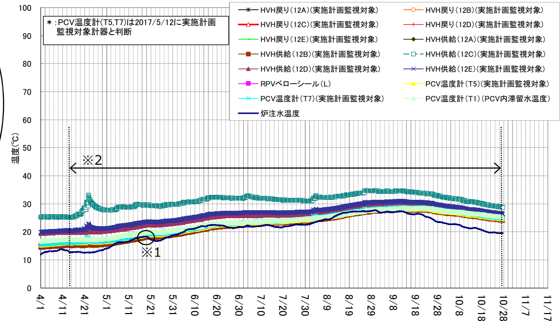
1号機 D/W雰囲気温度(4/1~10/27)
