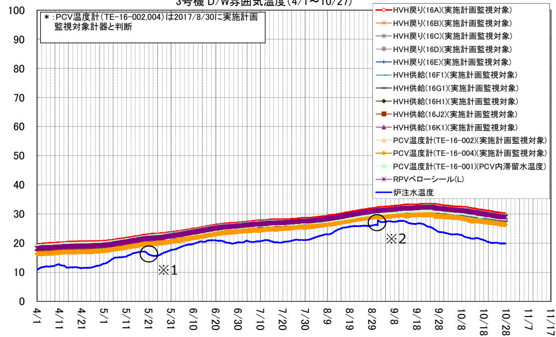
3号機 D/W雰囲気温度(4/1~10/27)
