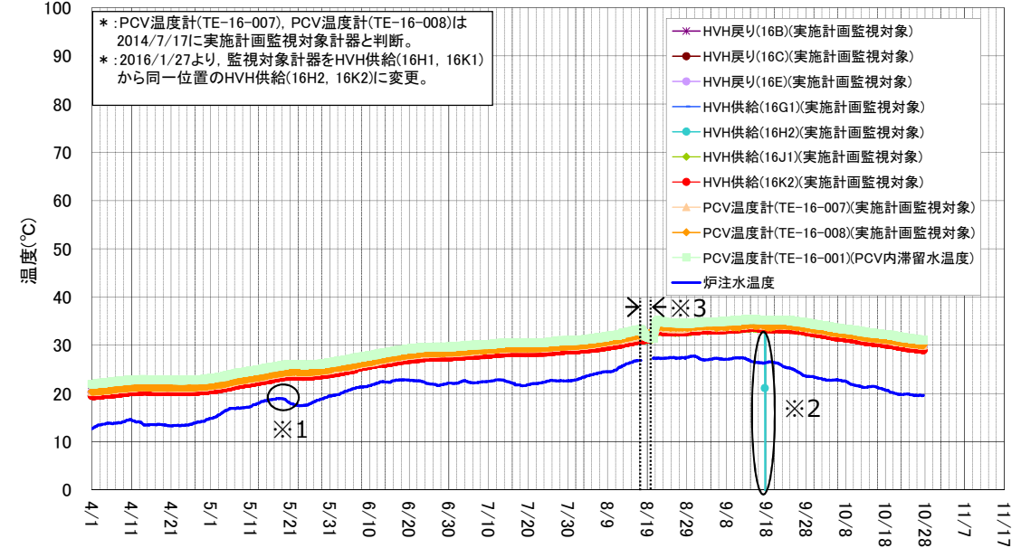
2号機 D/W雰囲気温度(4/1～10/27)
