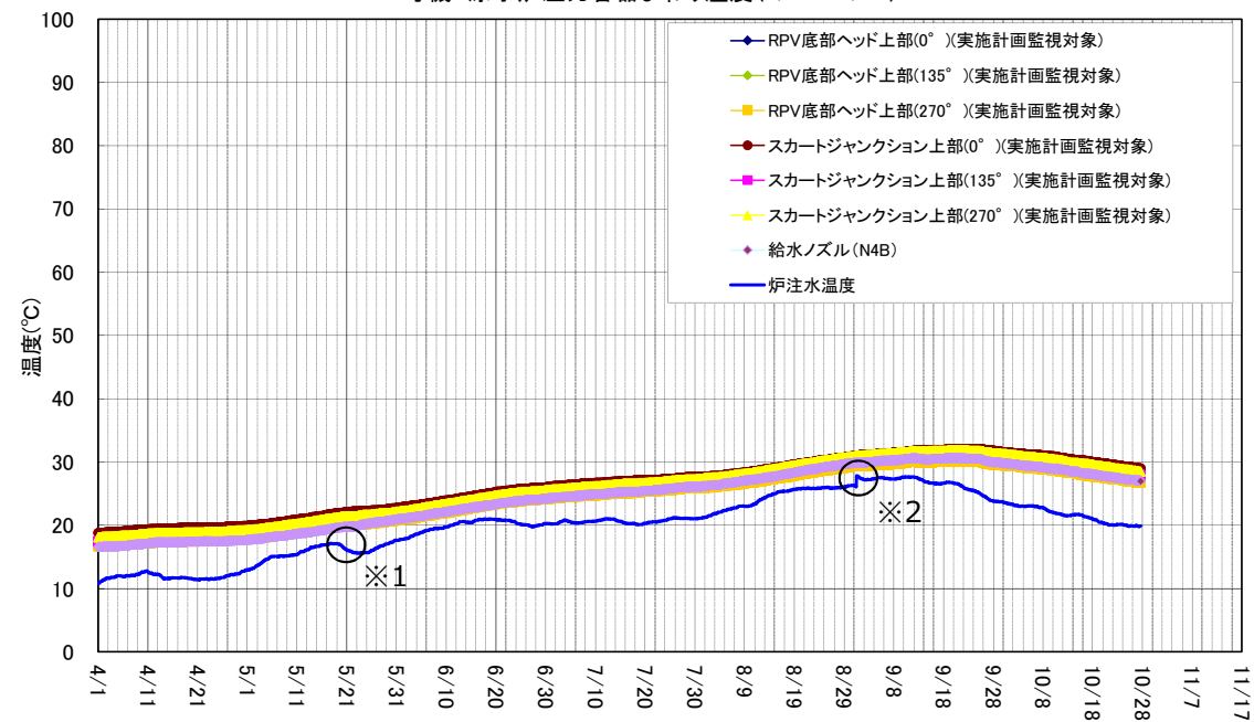
3号機 原子炉圧力容器まわり温度(4/1~10/27)
