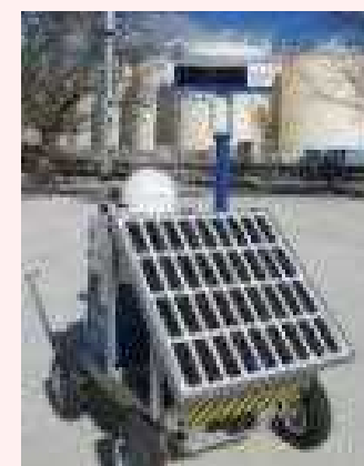
線量率モニタの設置状況
