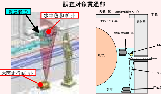
トラス室東側断面調査イメージ
