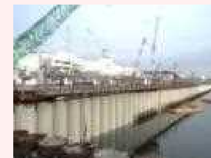
海側遮水壁 鋼管矢板打設完了状況
