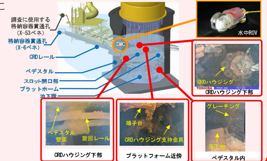
ペDESTAL内部の状況
