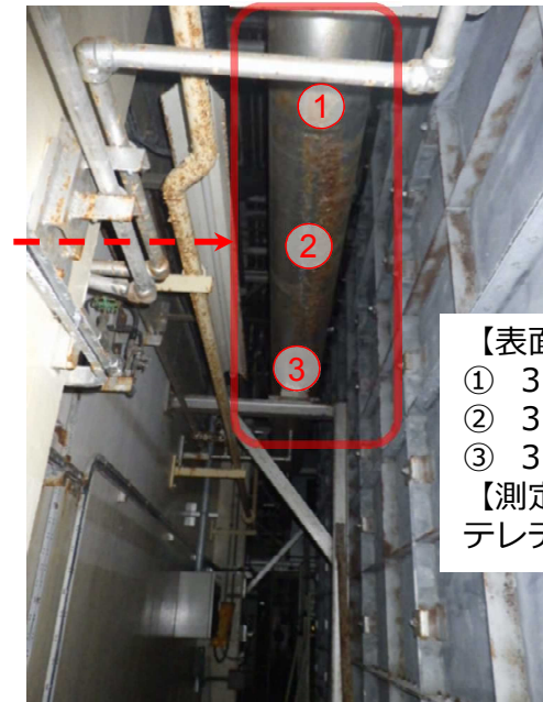
矢視(1)
