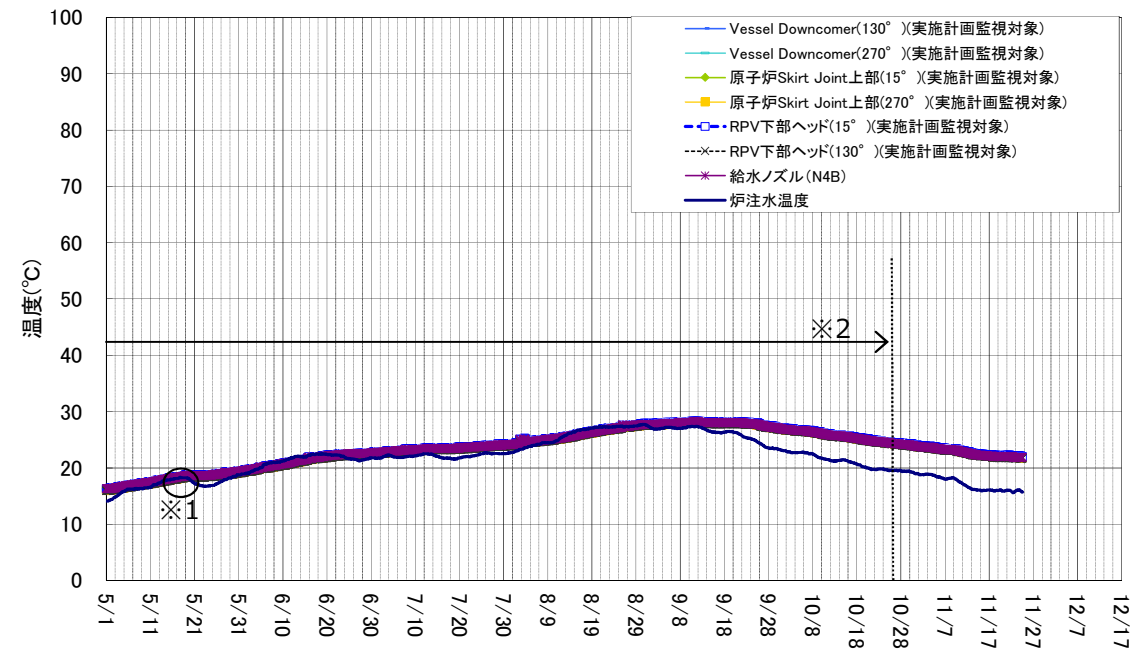
1号機 原子炉圧力容器まわり温度(5/1~11/24)
