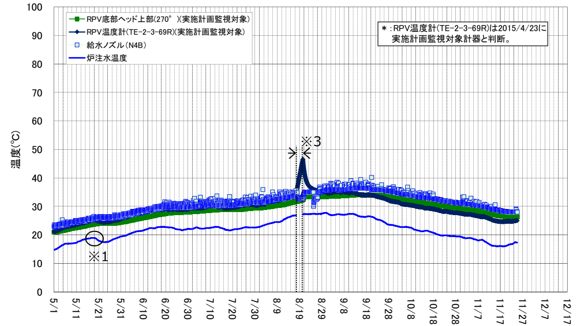
2号機 原子炉压力容器まわり温度 (5/1～11/24)
