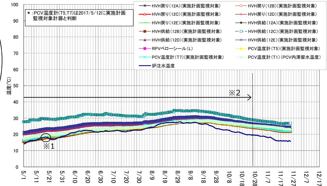
1号機 D/W雰囲気温度(5/1~11/24)
