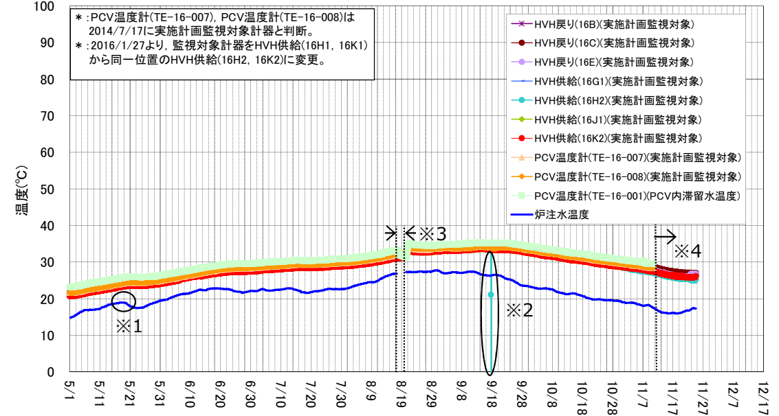
2号機 D/W雰囲気温度 (5/1～11/24)
