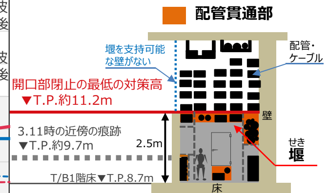
1R-1'堰（対策断面イメージ）
