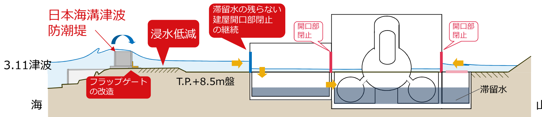
※1～4号機断面イメージ
