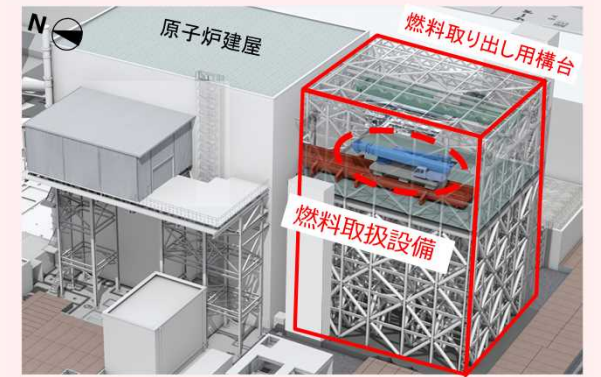
燃料取り出し概要図(鳥瞰図)
