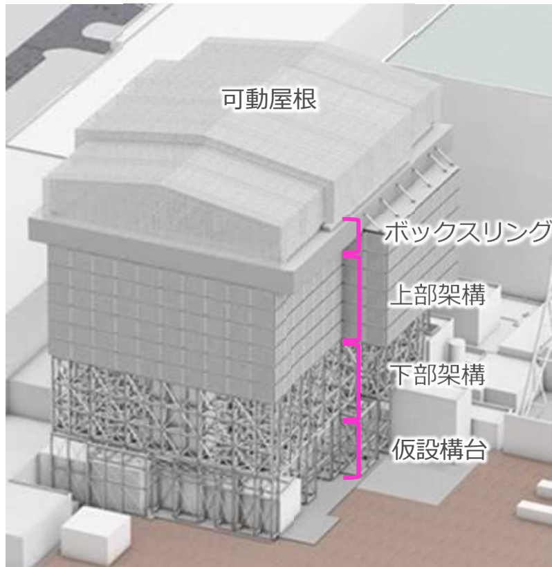
大型カバー全体の概要図
