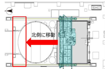
③干渉物撤去 (FHM移動) ※2
