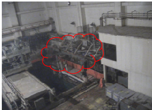
⑤干渉物撤去 (SFP南側既設設備撤去) ※4
