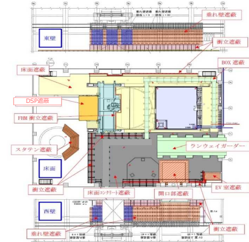
⑦遮蔽設置 (その2)
