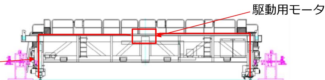
カップリング切断装置配置図
