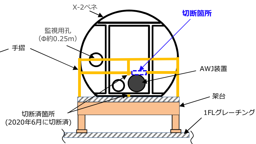
断面図による切断イメージ (紙面手前側が原子炉圧力容器)
