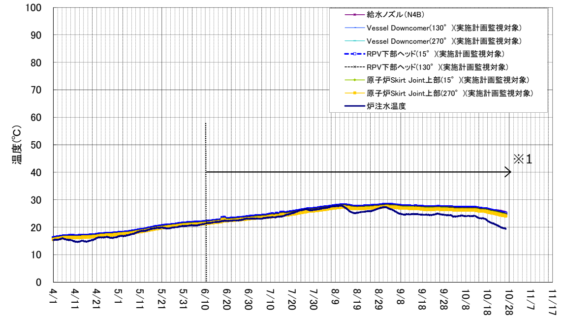
1号機 原子炉圧力容器まわり温度(4/1~10/26)
