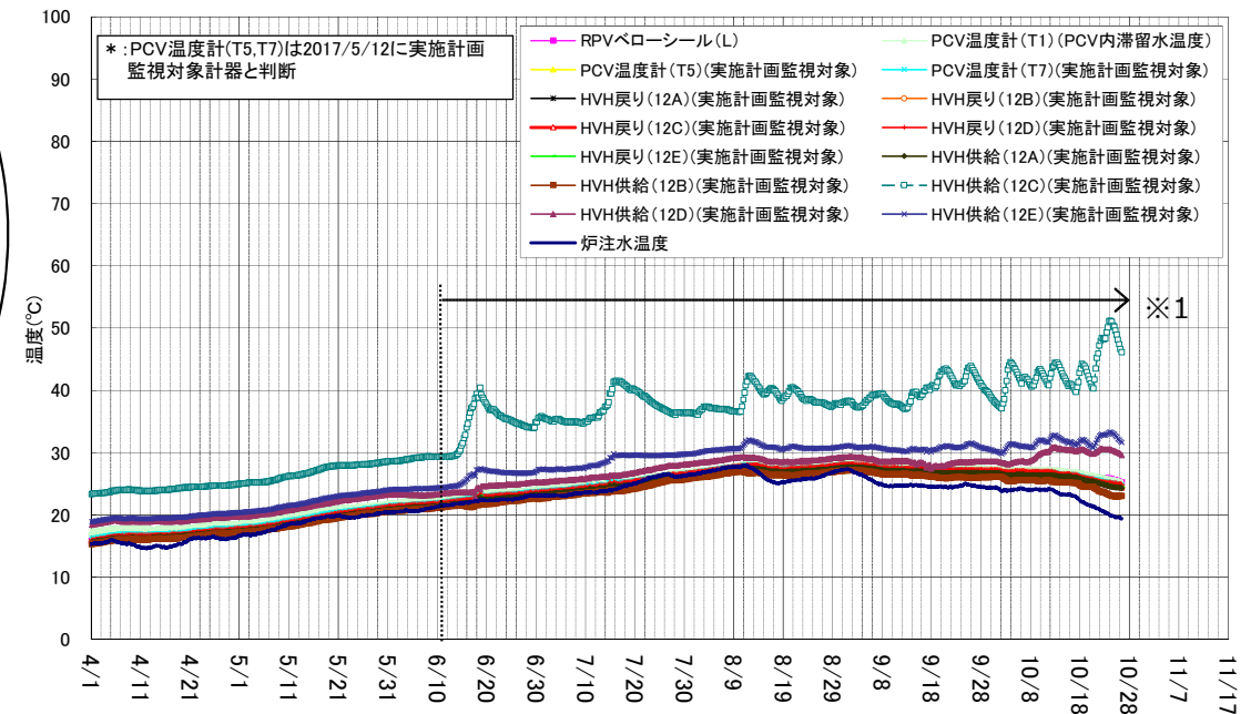
1号機 D/W雰囲気温度(4/1~10/26)
