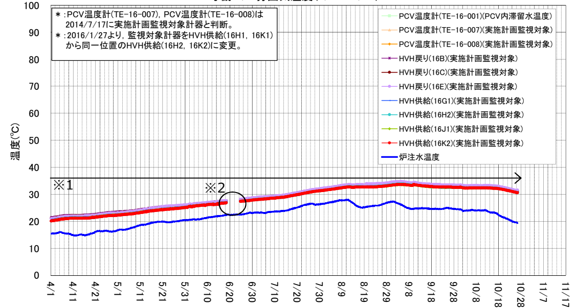
2号機 D/W雰囲気温度 (4/1～10/26)
