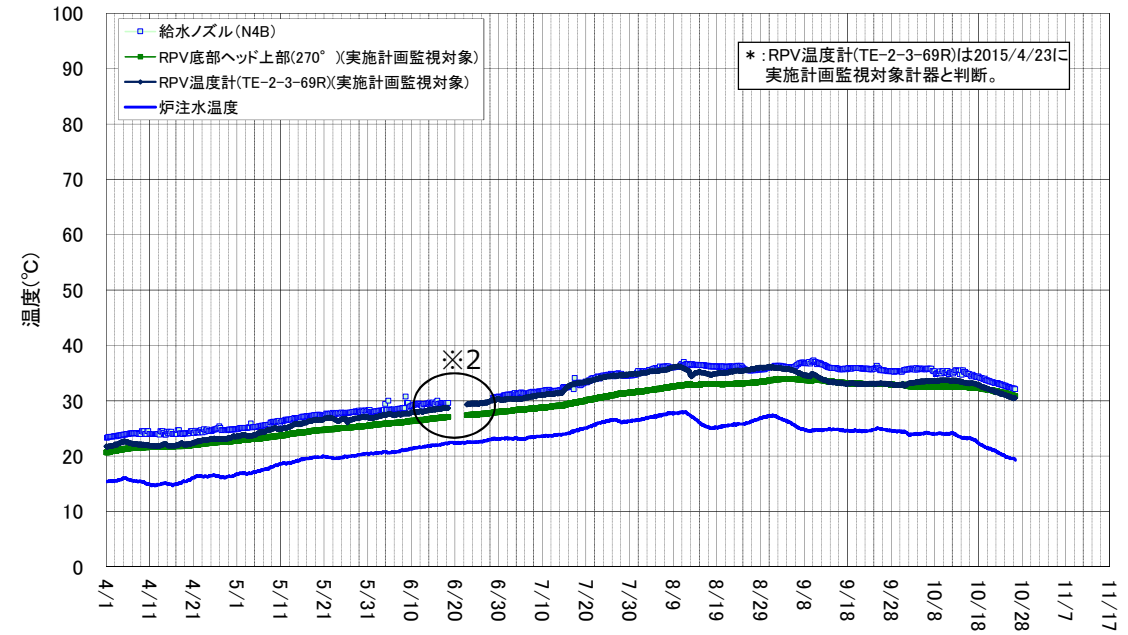
2号機 原子炉圧力容器まわり温度 (4/1～10/26)
