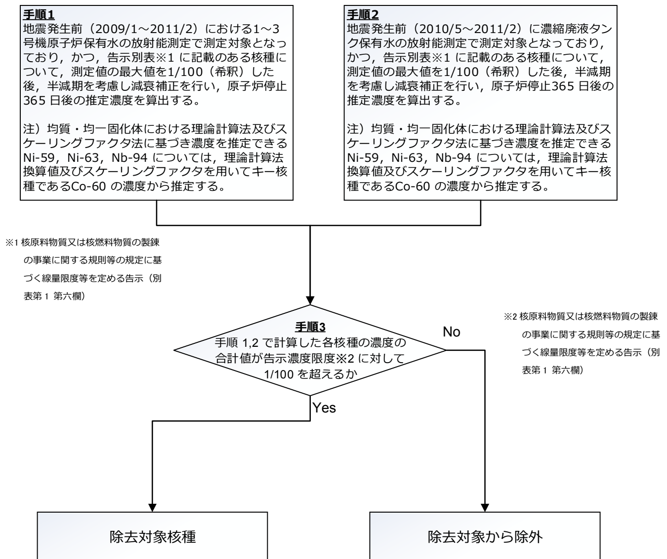
図 C - 2 CP 核種における除去対象核種選定フロー
