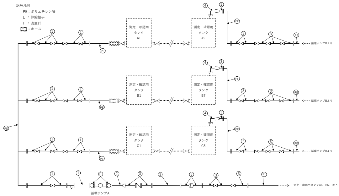
図－１ 配管概略図（１／４） （測定・確認用設備）
