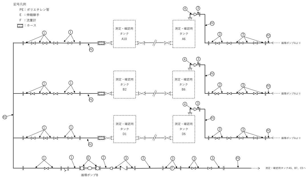
図－２ 配管概略図（２／４） （測定・確認用設備）
