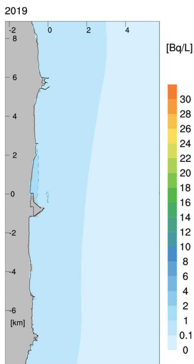
図 F - 3 放水位置の違いによる海表面の年間平均濃度分布図の比較 (拡大図)
