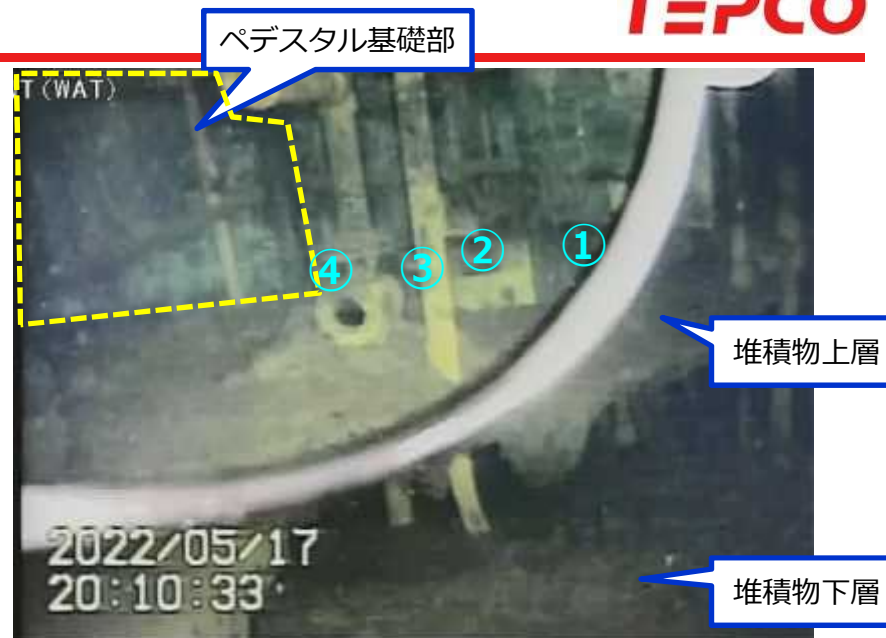
写真1.ペDESTアル基礎部(上部)の状況
