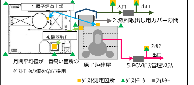
3号機原子炉建屋の開口部のイメージ 月間平均値が一番高い箇所の ■ダスト測定箇所 ▲ダストモニタ ■フィルター
