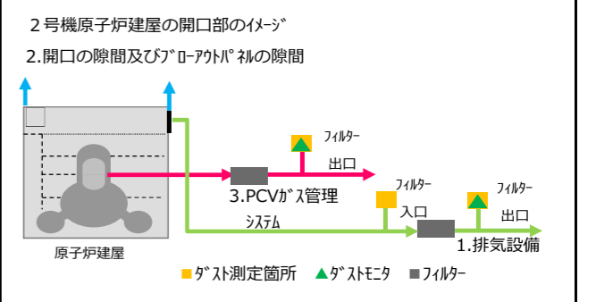
2号機原子炉建屋の開口部のイメージ 2. 開口の隙間及びBOPの隙間 ■ダスト測定箇所 ▲ダストモニタ ■フィルター
