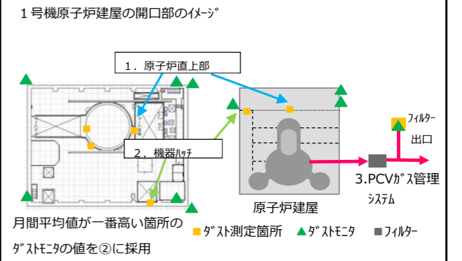
1号機原子炉建屋の開口部のイメージ 月間平均値が一番高い箇所の ■ダスト測定箇所 ▲ダストモニタ ■フィルター ダストモニタの値を②に採用
