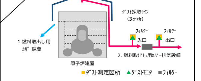
4号機原子炉建屋の開口部のイメージ ダスト採取ポイント(3ヶ所) ■ダスト測定箇所 ▲ダストモニタ ■フィルター
