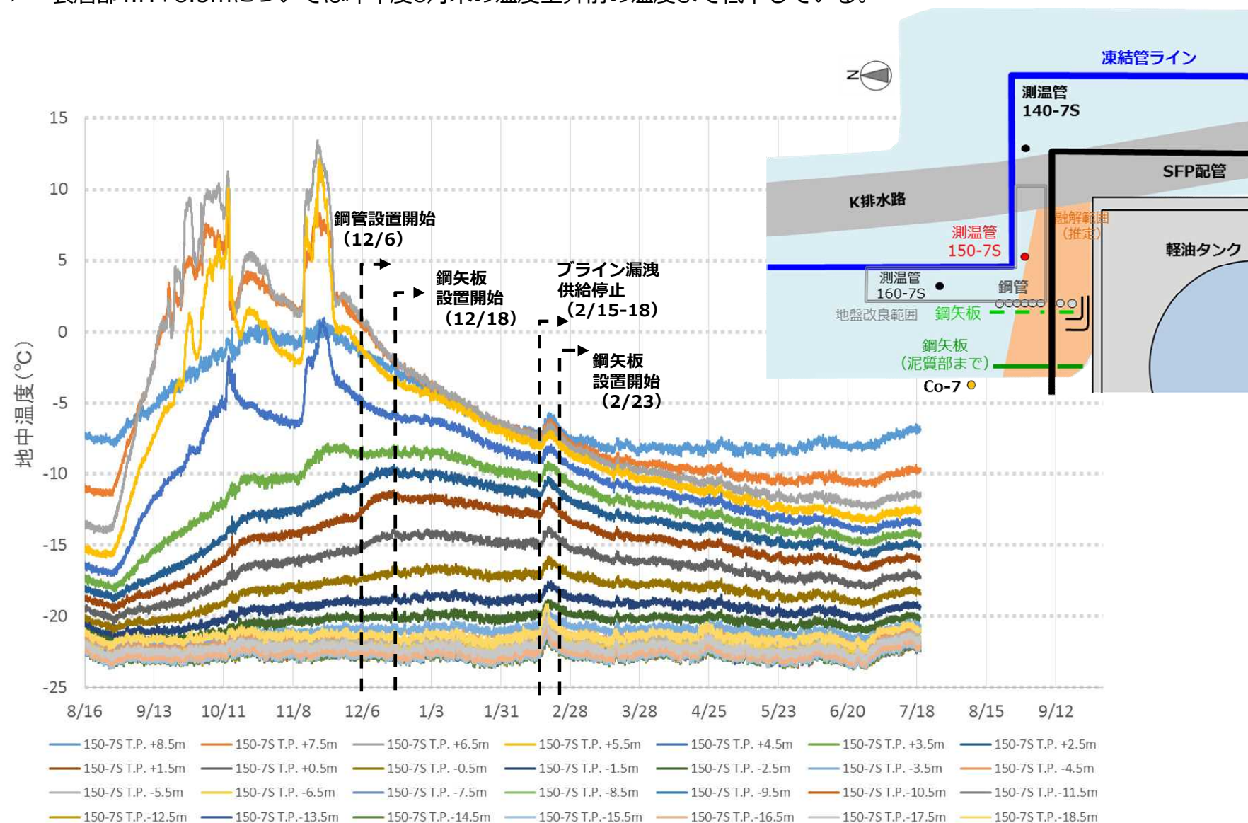
測温管150-7S経時変化 (7/19 7:00時点)
