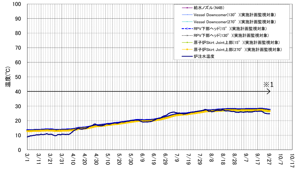
1号機 原子炉圧力容器まわり温度(3/1~9/27)
