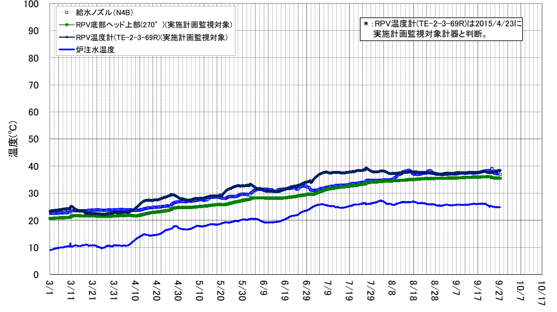
2号機 原子炉圧力容器まわり温度(3/1~9/27)
