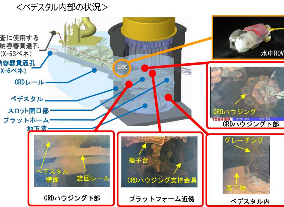
3号機 PCV内部調査実績
