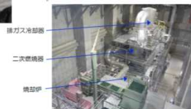
雑固体廃棄物焼却設備 焼却設備全体（写真左：A系 右：B系）
