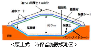
＜覆土式一時保管施設概略図＞
