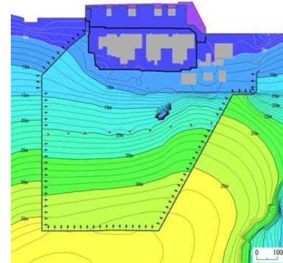
現況 + 広域遮水壁及び集水井
