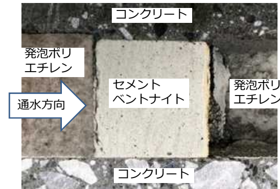
(3) セメントベントナイト 水中打設の切断面
