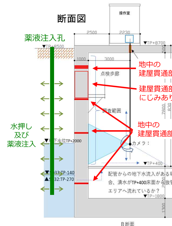
B断面
