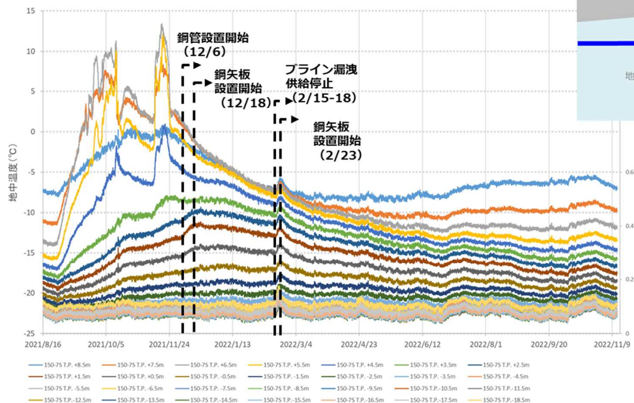
測温管150-7 S 経時変化 (11/15 19:00時点)
