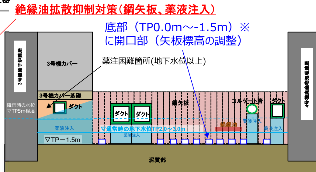
断面図(a-a)
