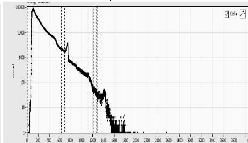
【γ線測定】
