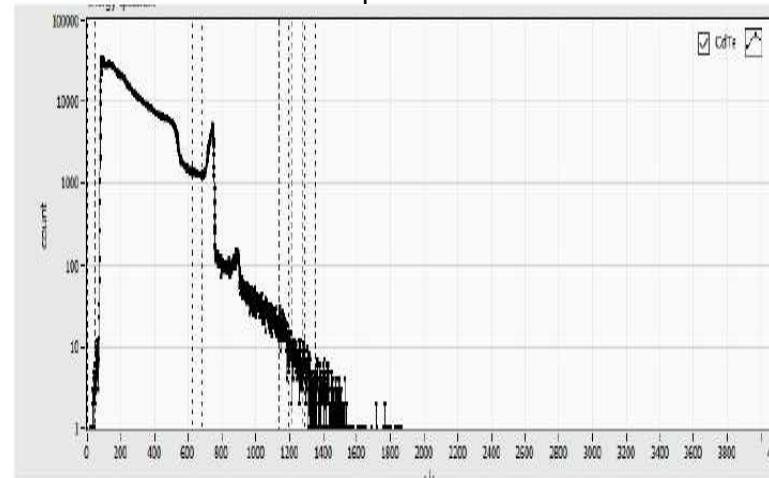
【γ線測定】
