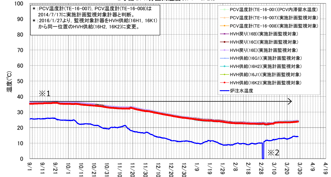
2号機 D/W雰囲気温度(9/1～3/28)
