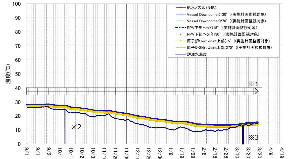
1号機 原子炉圧力容器まわり温度 (9/1~3/28)
