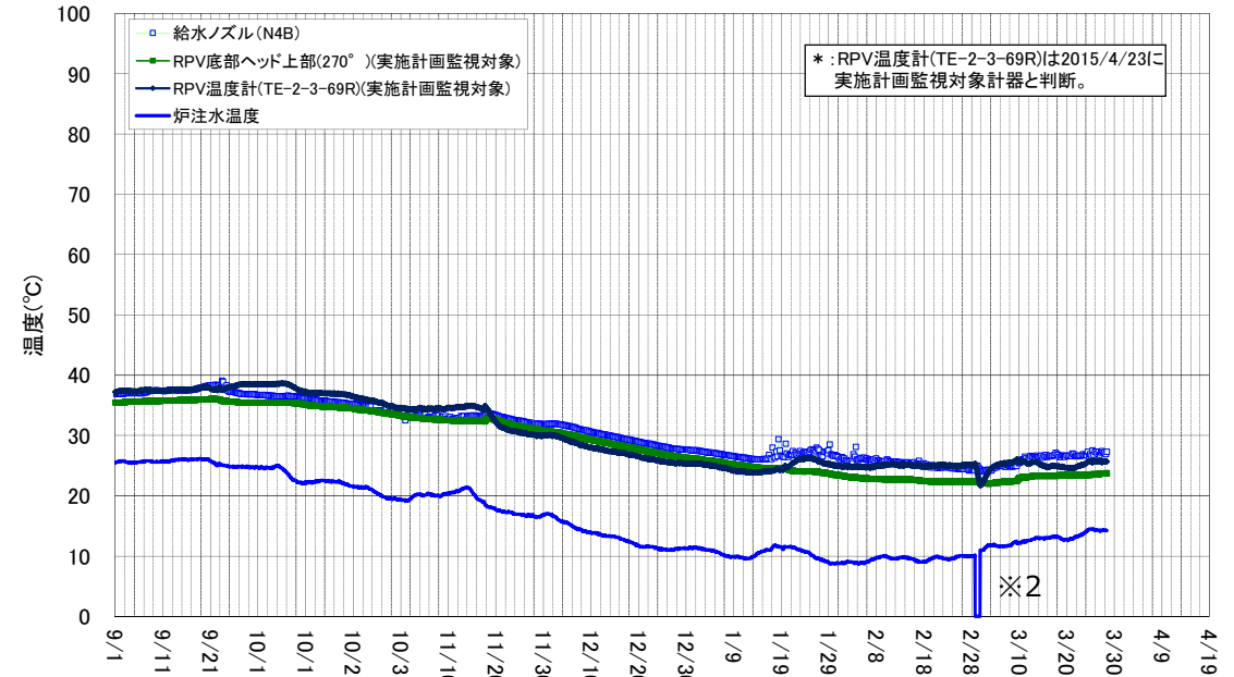
2号機 原子炉圧力容器まわり温度(9/1～3/28)
