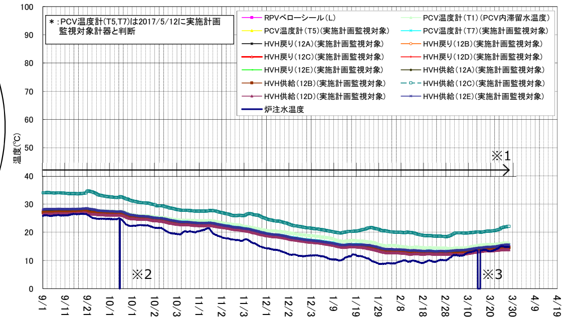
1号機 D/W雰囲気温度 (9/1~3/28)
