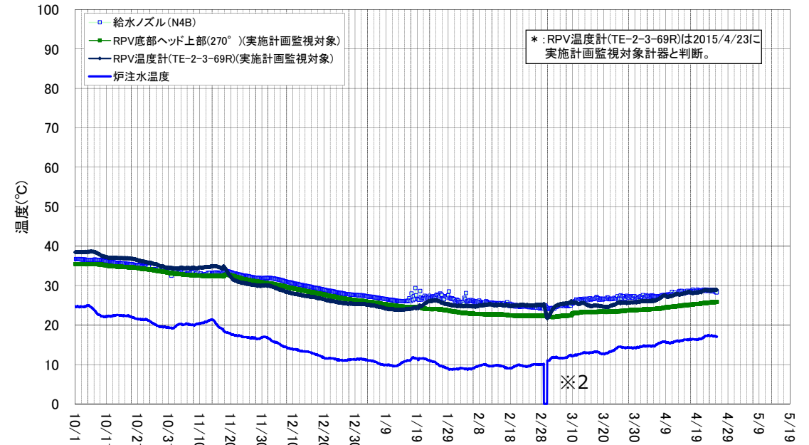
2号機 原子炉圧力容器まわり温度(10/1～4/25)
