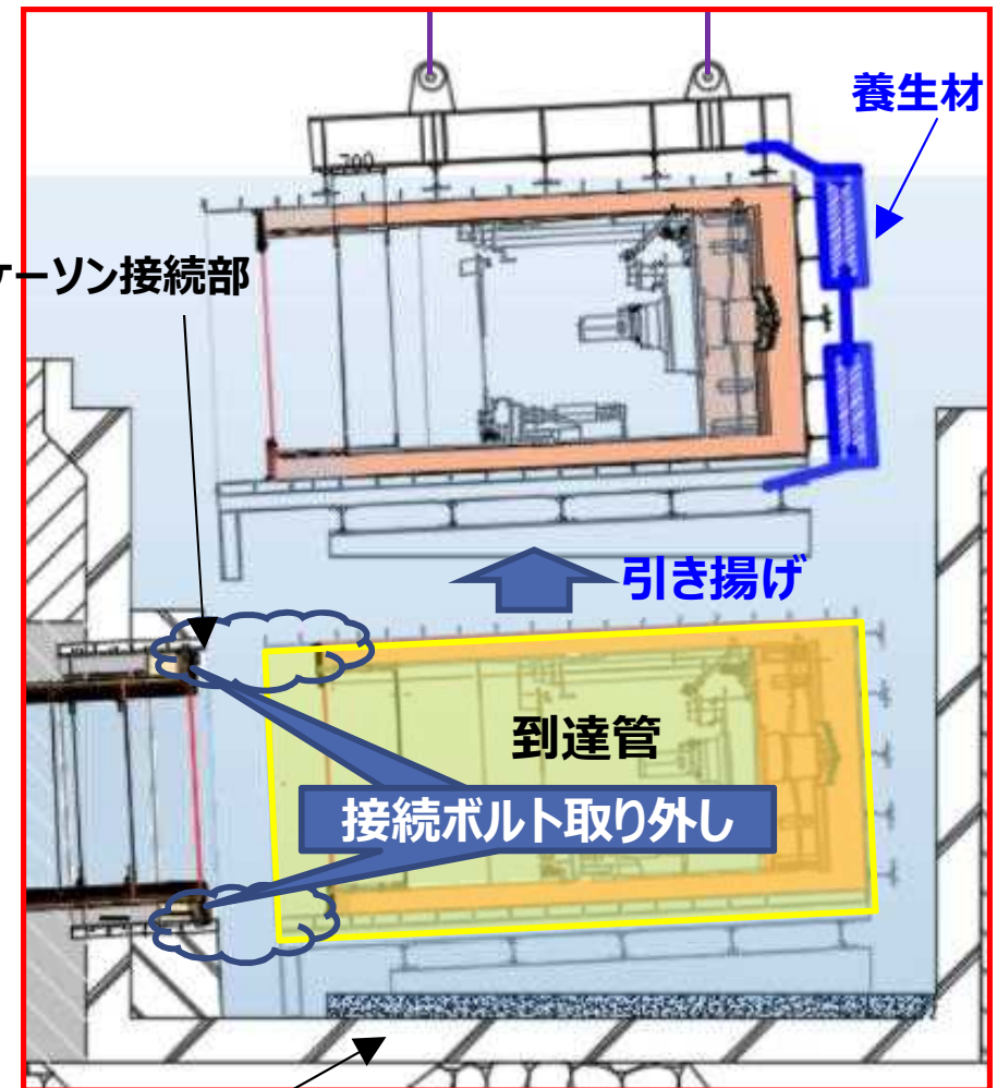
放水口ケーソン
