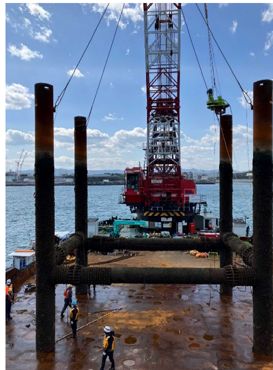
測量櫓（上段）撤去状況
