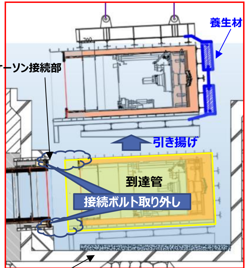
放水口ケーソン
