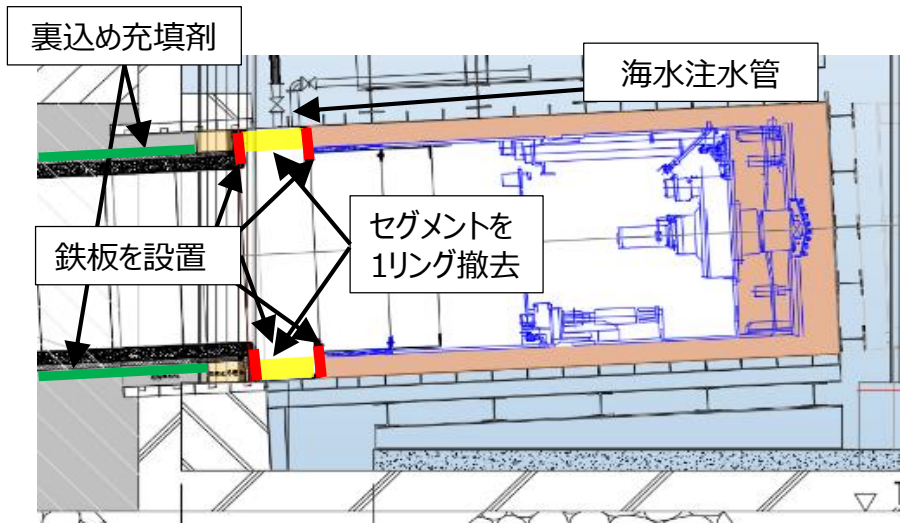
止水工事 イメージ図
