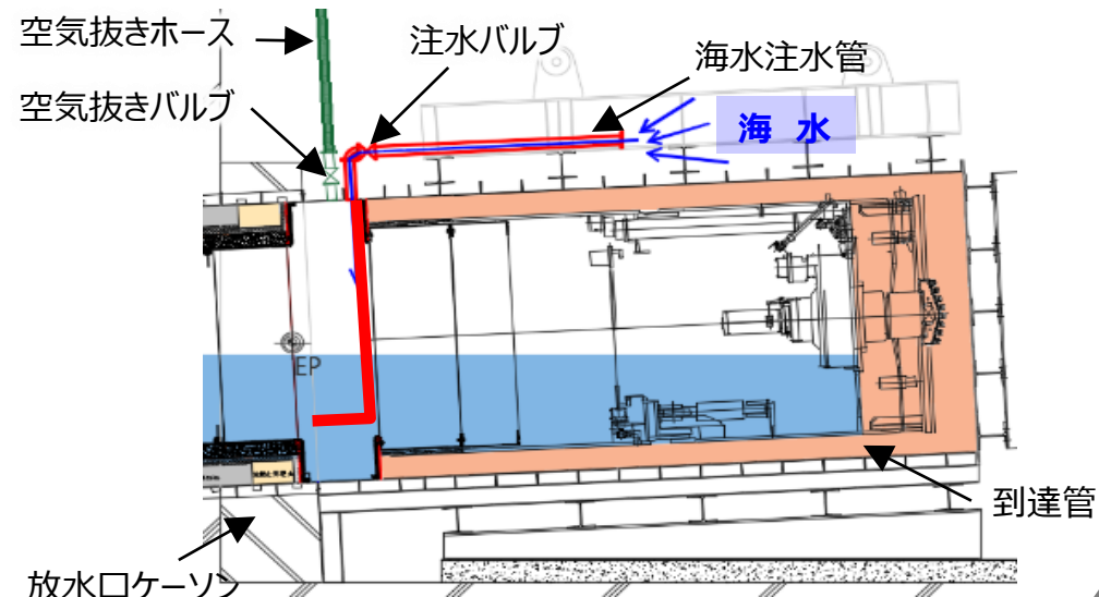
海水注入 イメージ図
