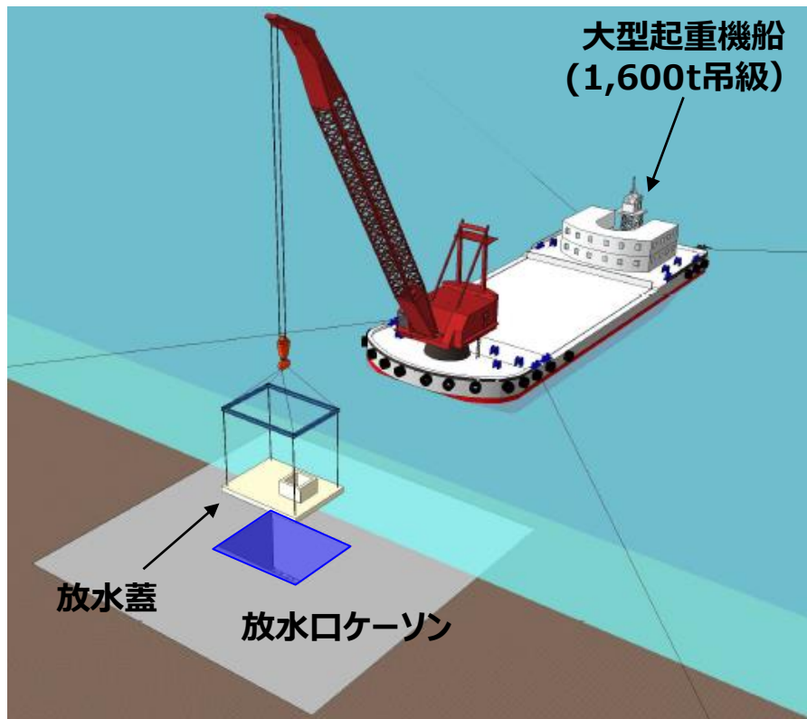
放水蓋据付イメージ図
